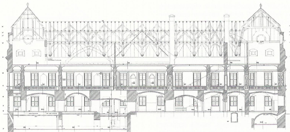
Az északi szárny hosszmetsete
