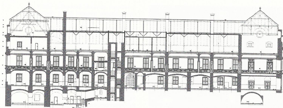
A nyugati szárny hosszmetsete (a szerző rajzai)
