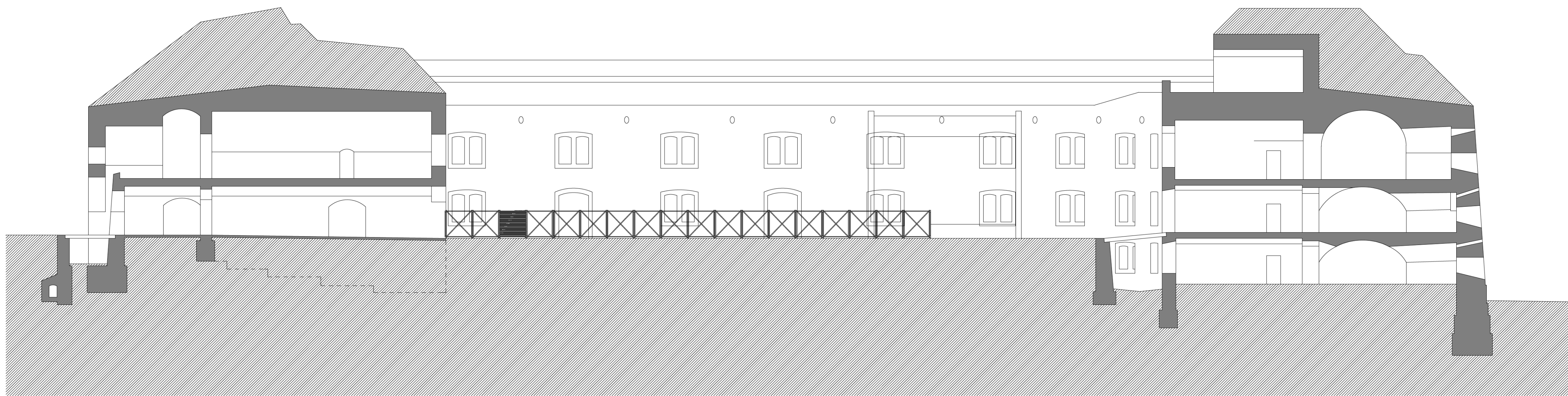
A-A METSZET
