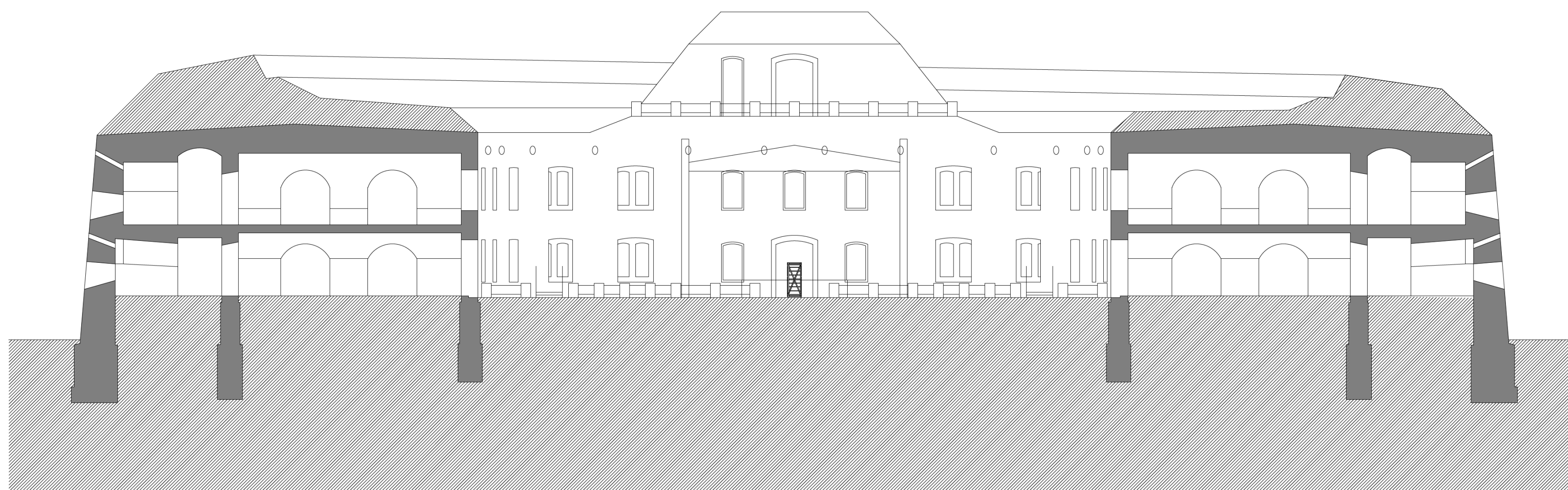
B-B METSZET
