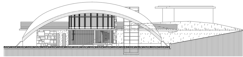
keleti homlokzat
