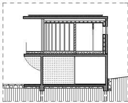
a-a metszet
