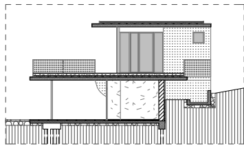
b-b metszet
