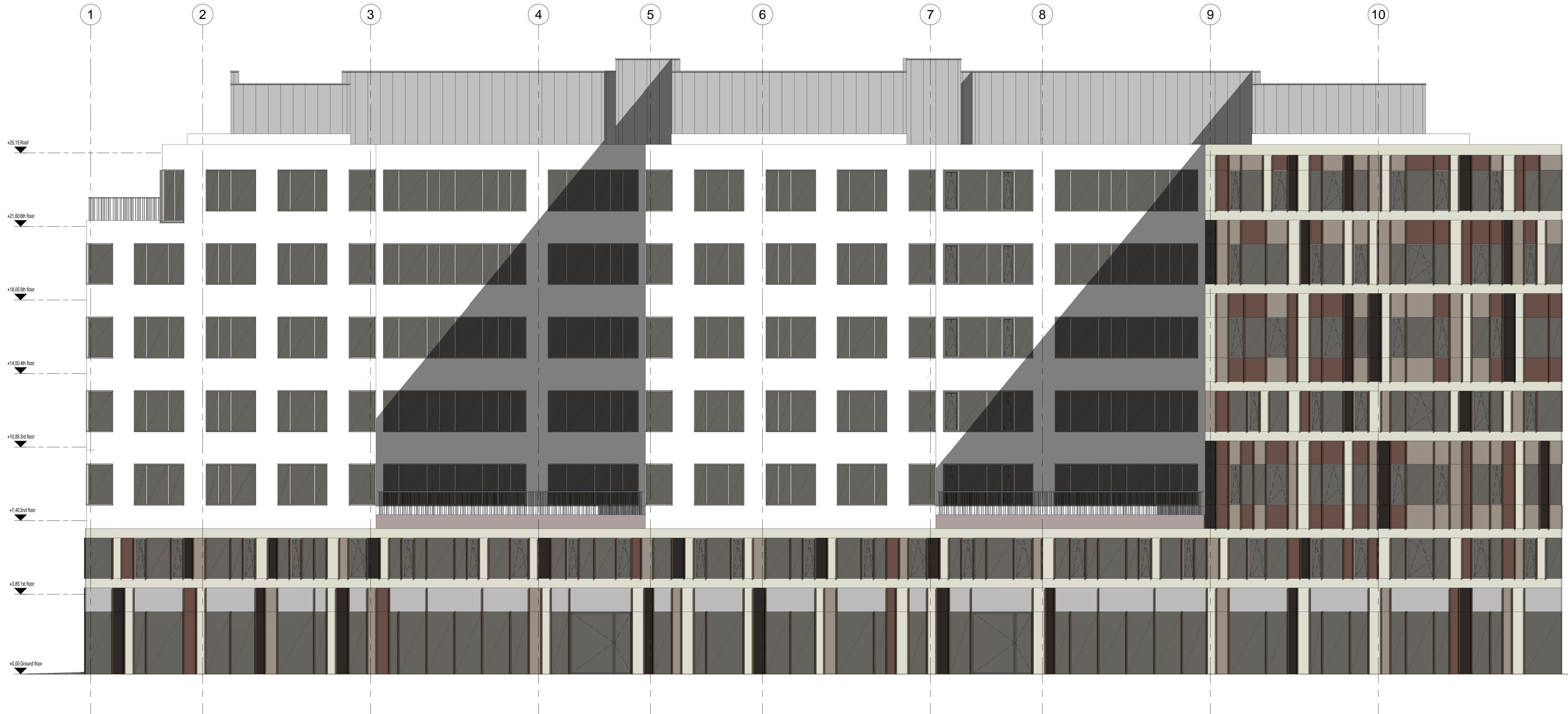
Fiastyúk utca Facade M1 Scale 1 : 100
