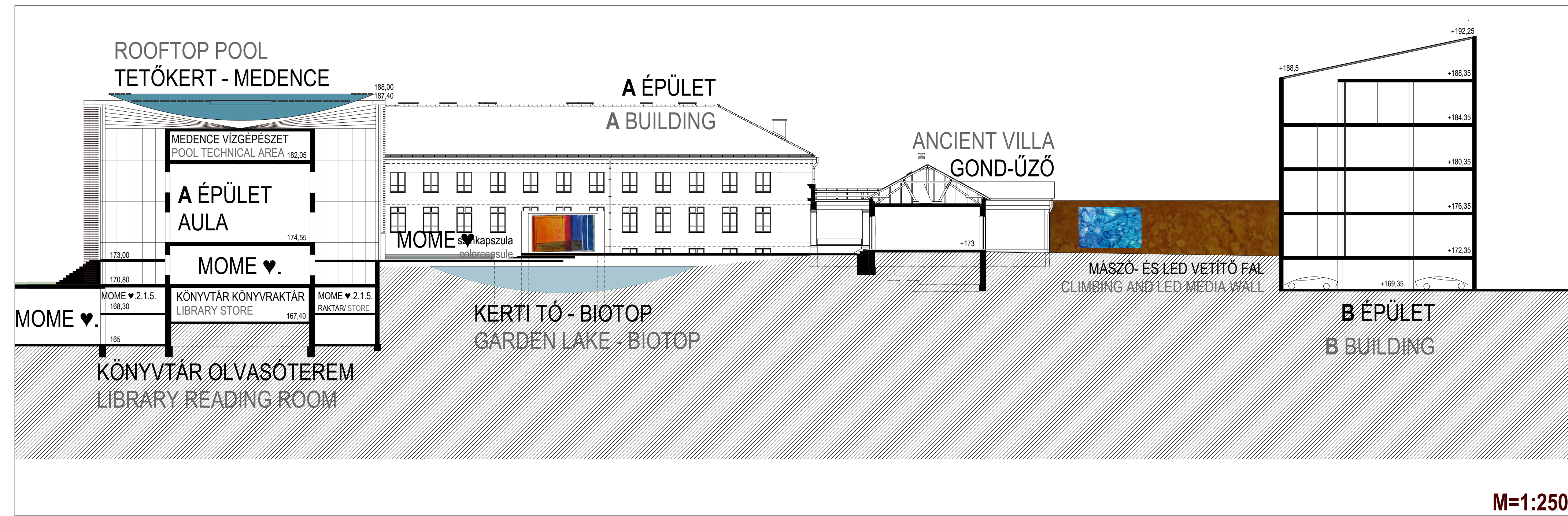
METSZET A KÖNYVTÁRON ÉS A B ÉPÜLETEN ÁT/ SECTION ACROSS THE LIBRARY AND THE B BUILDING
