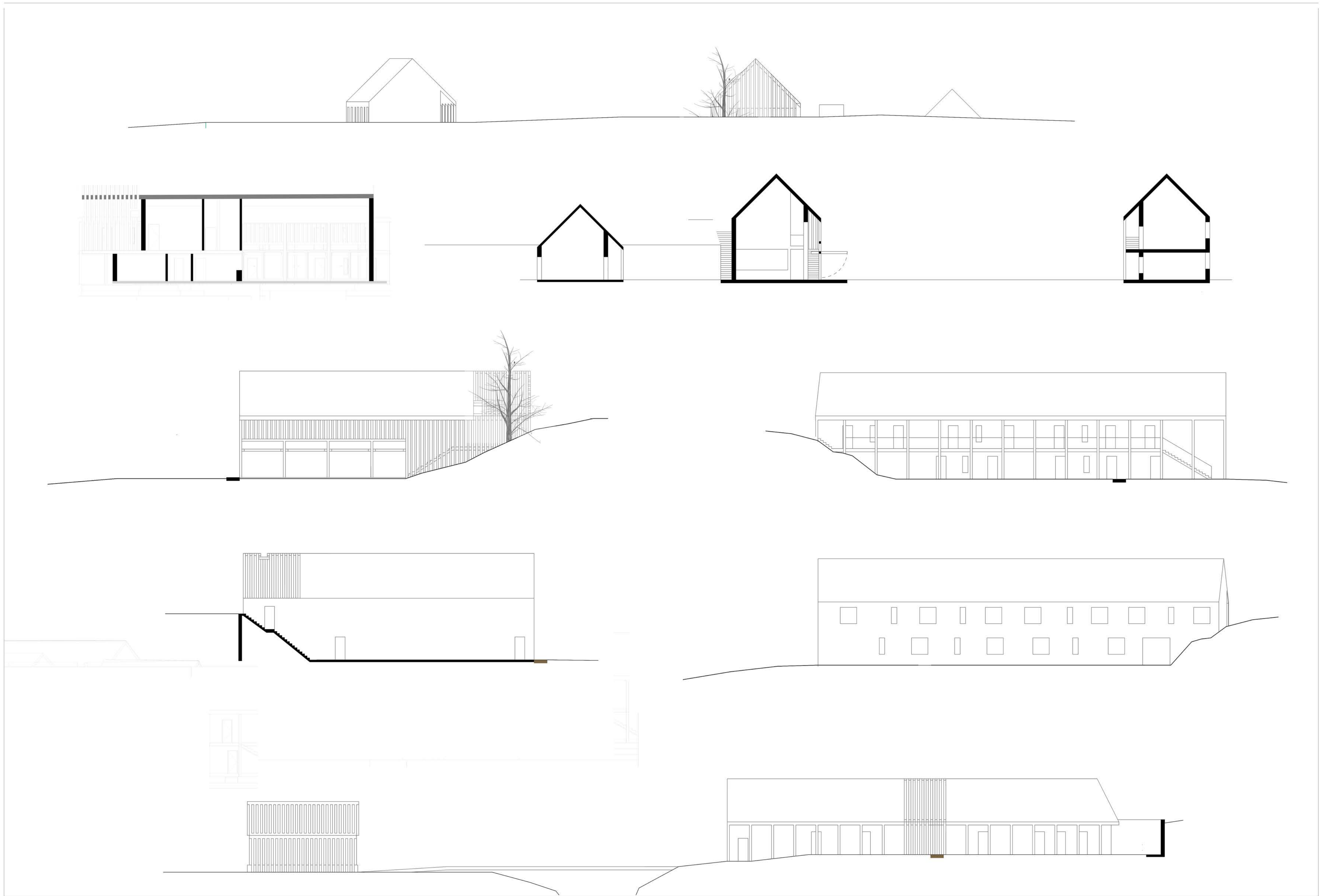
M 1:200 Homlokzatok és metszetek
