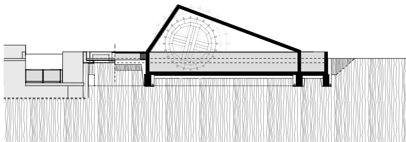
a-a metszet
