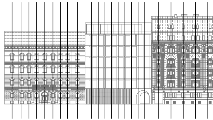
UTCAI HOMLOKZAT VERTIKÁLIS RITMUSA
