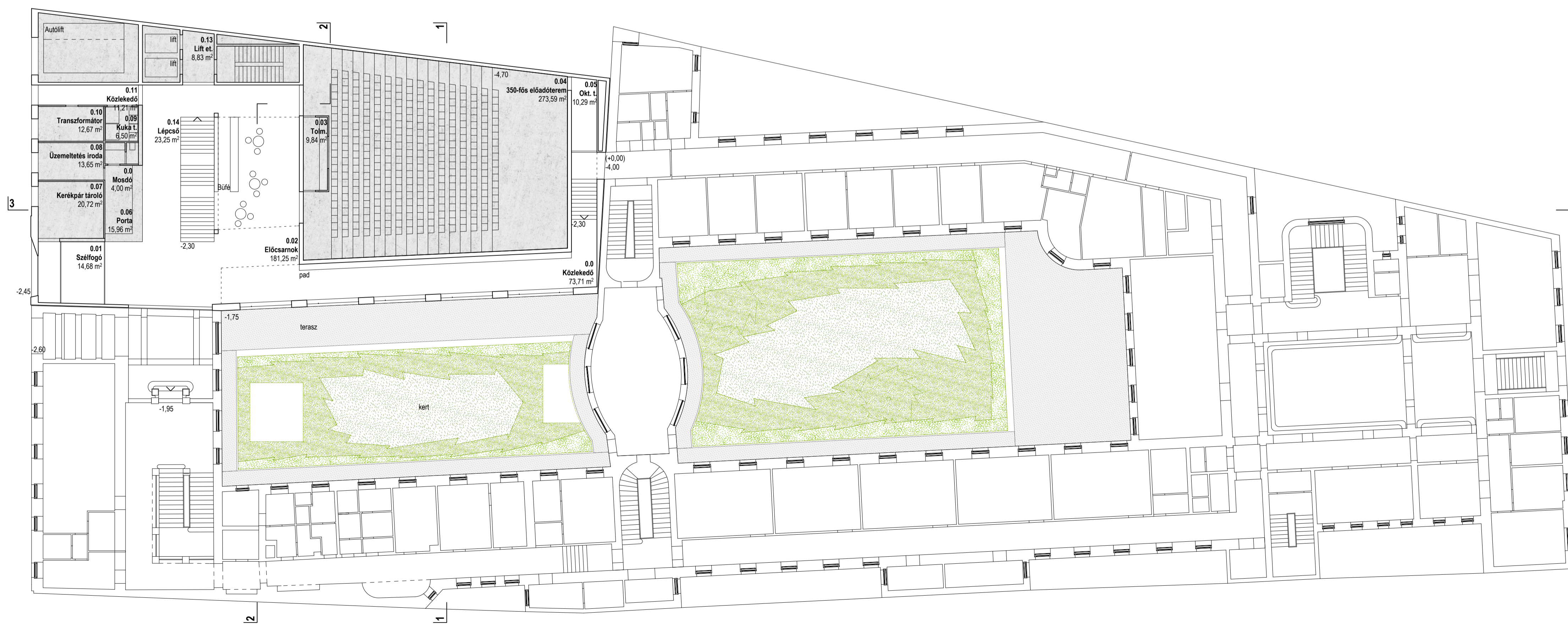
Földszinti alaprajz M 1:200
