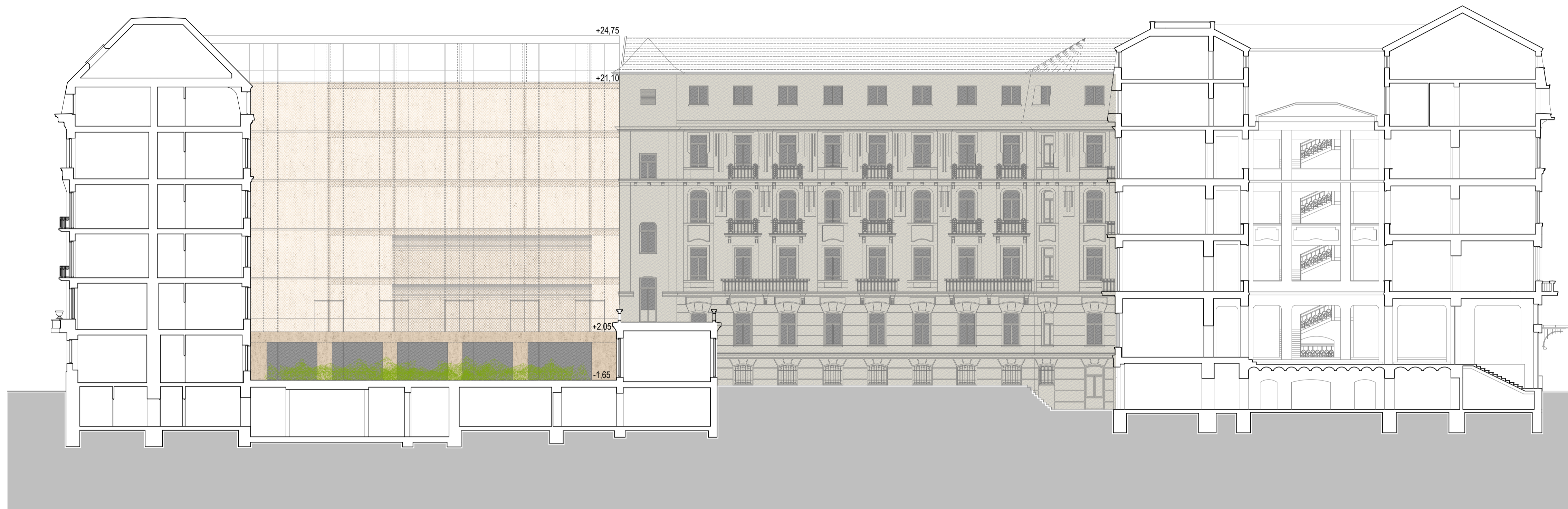
Udvari homlokzat M 1:200
