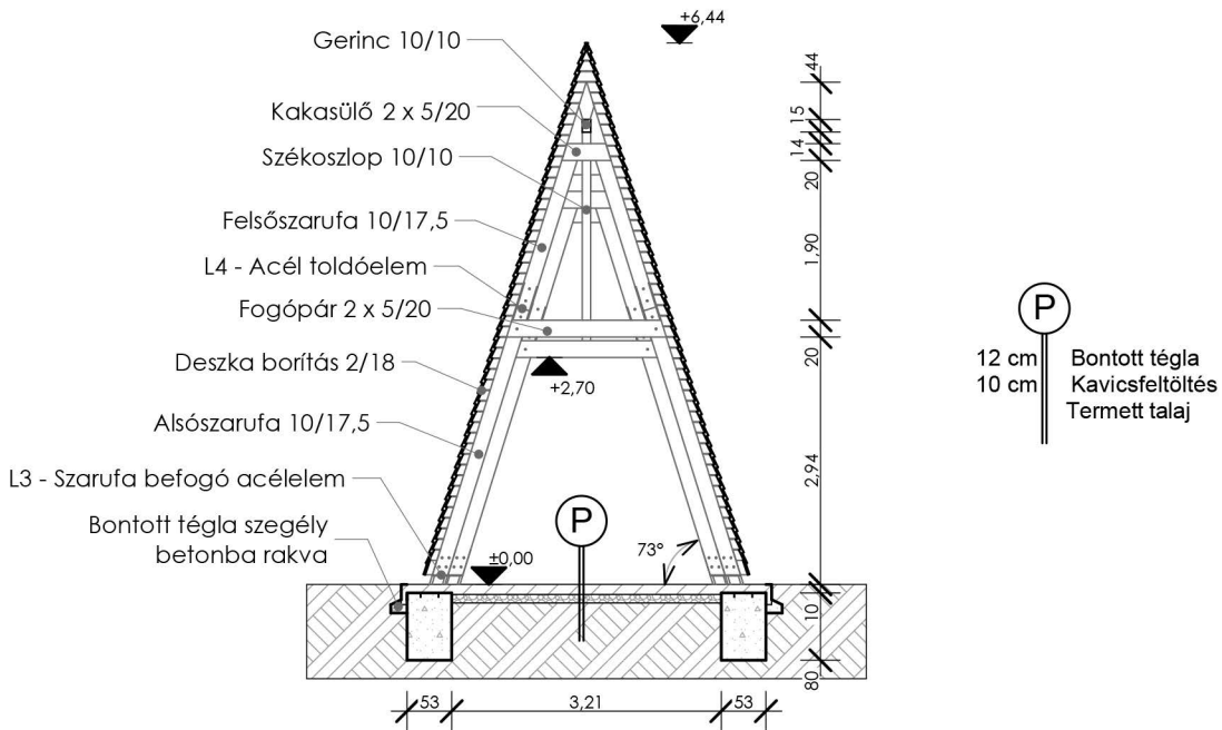
TEMETŐ EMLÉKHELY A-A METSZET, m= 1:100
