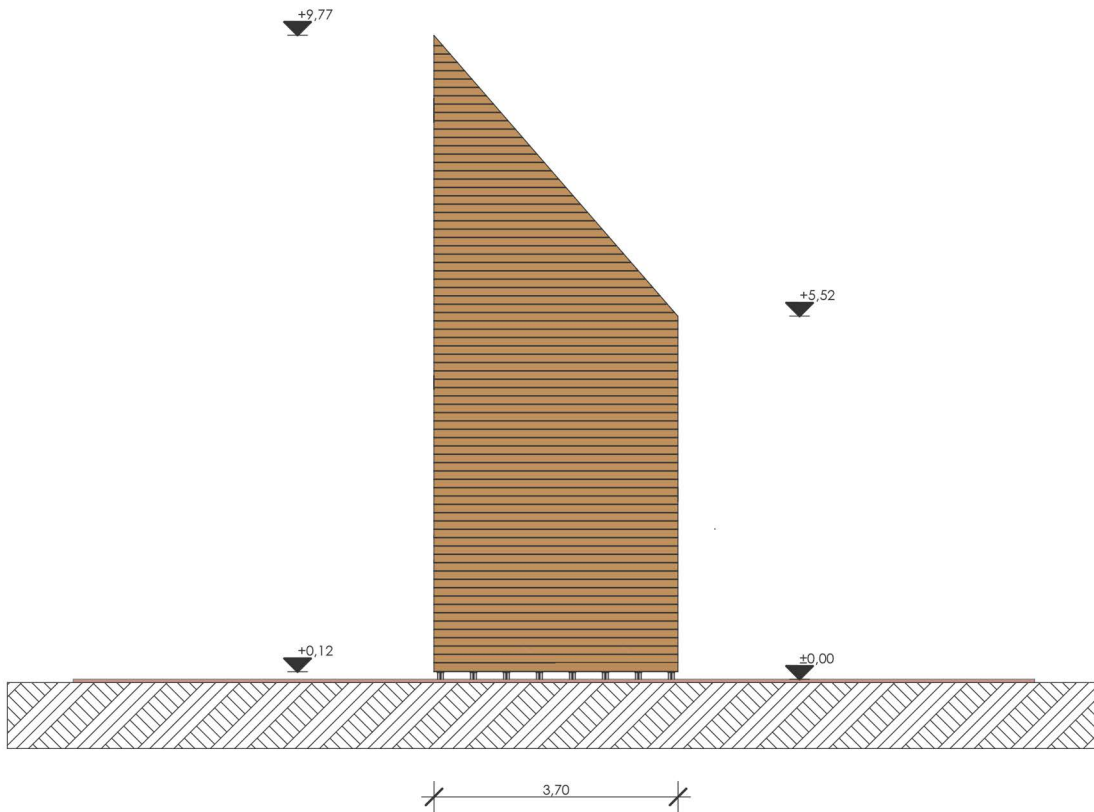
TEMETŐ EMLÉKHELY DÉLI HOMLOKZAT, m= 1:100
