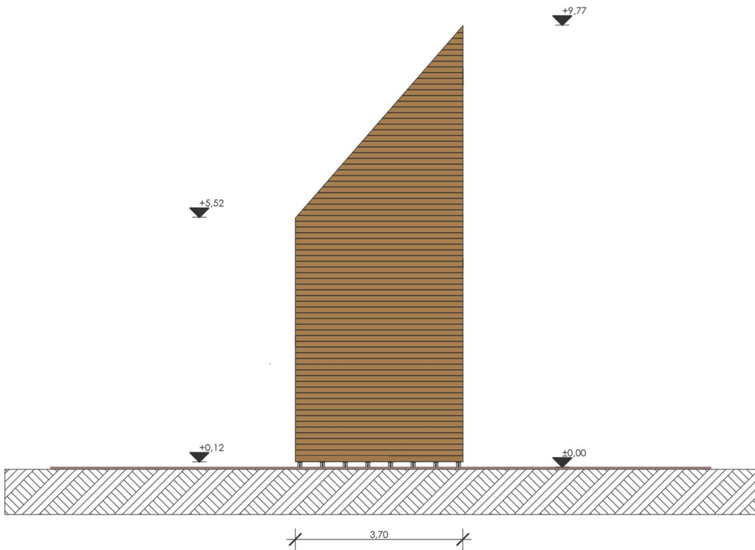
TEMETŐ EMLÉKHELY ÉSZAKI HOMLKZAT, m= 1:100
