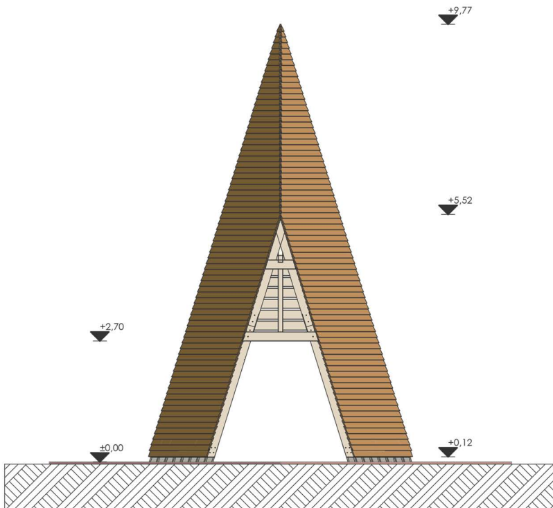
TEMETŐ EMLÉKHELY NYUGATI HOMLOKZAT, m= 1:100
