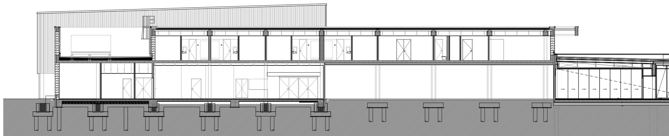
C - C METSZET
