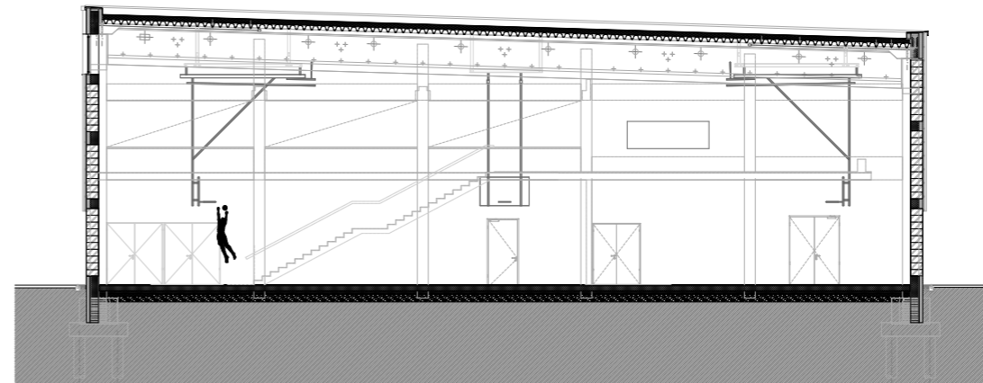
A - A METSZET
