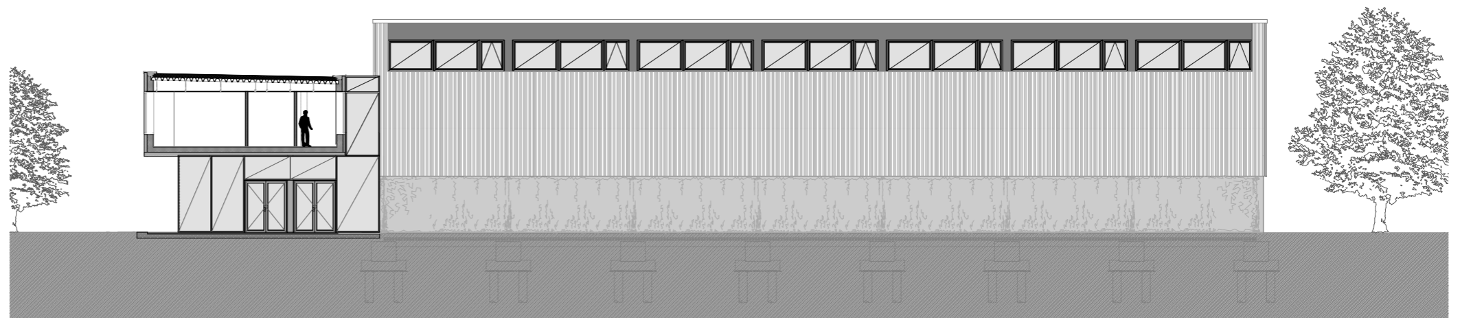
ÉSZAKNYUGATI HOMLOKZAT
