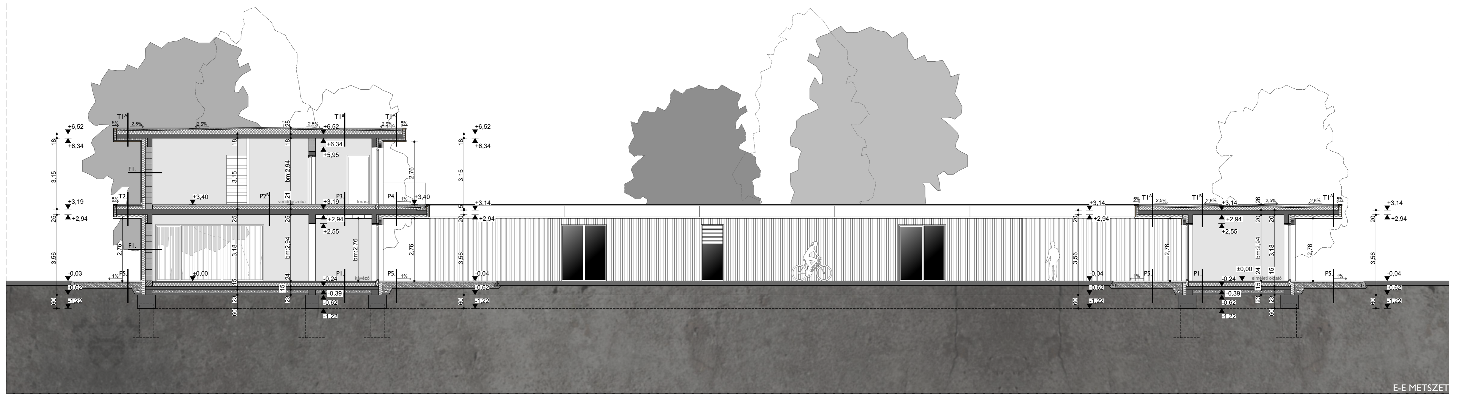
E-E METSZET
