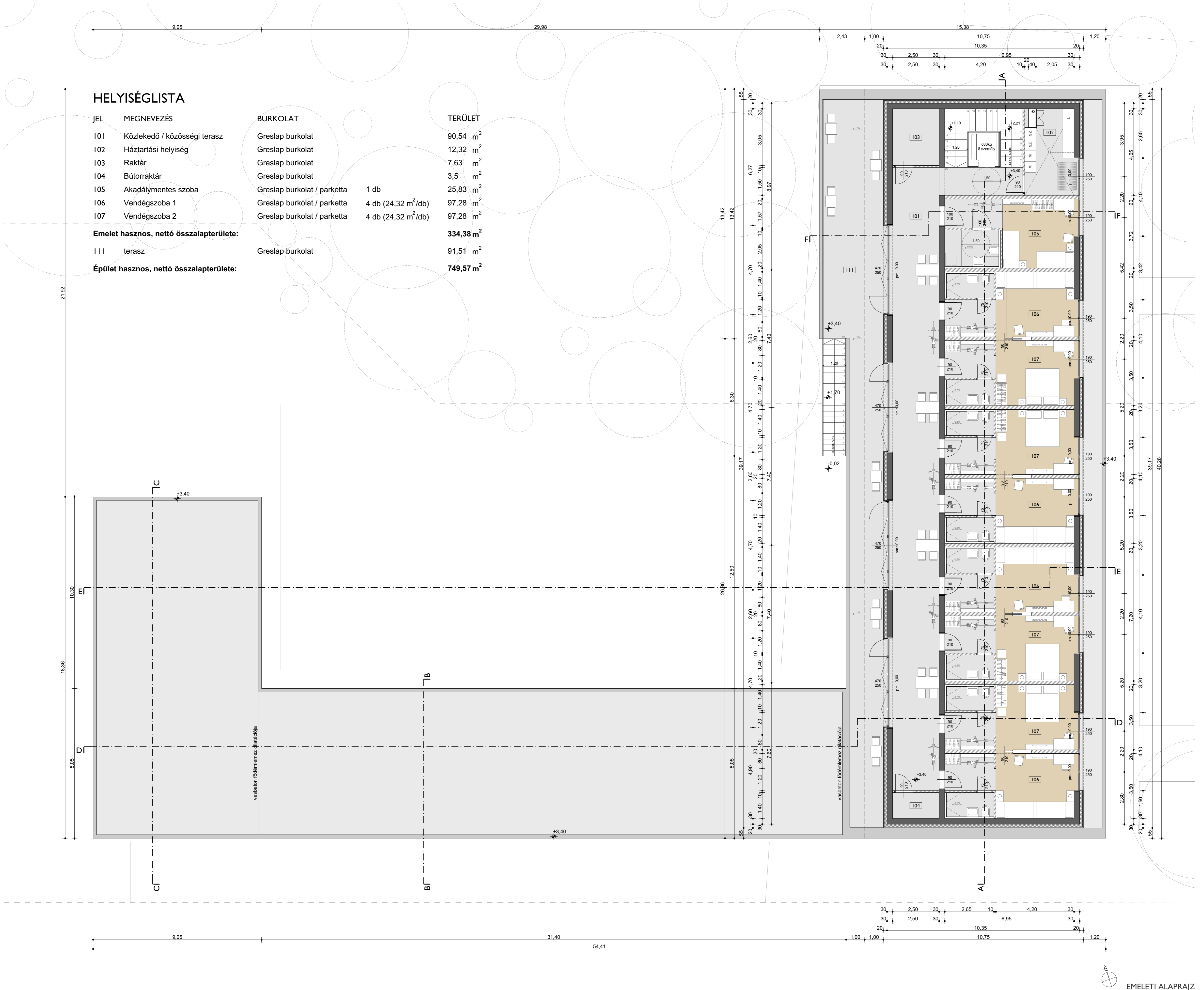
EMELET ALAPRAJZ
