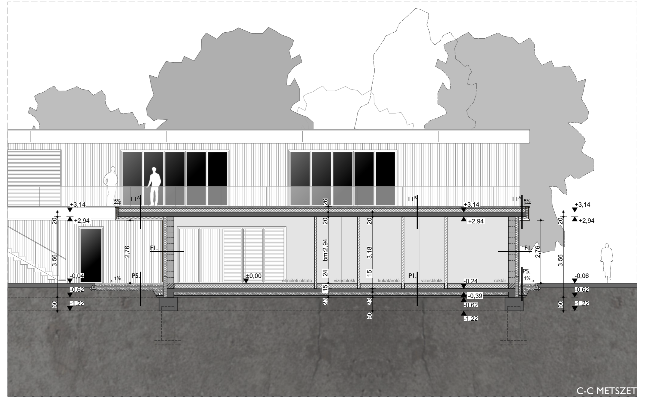
C-C METSZET
