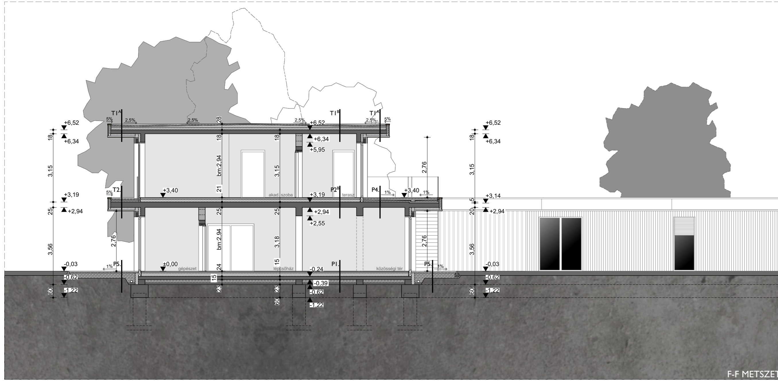
F-F METSZET
