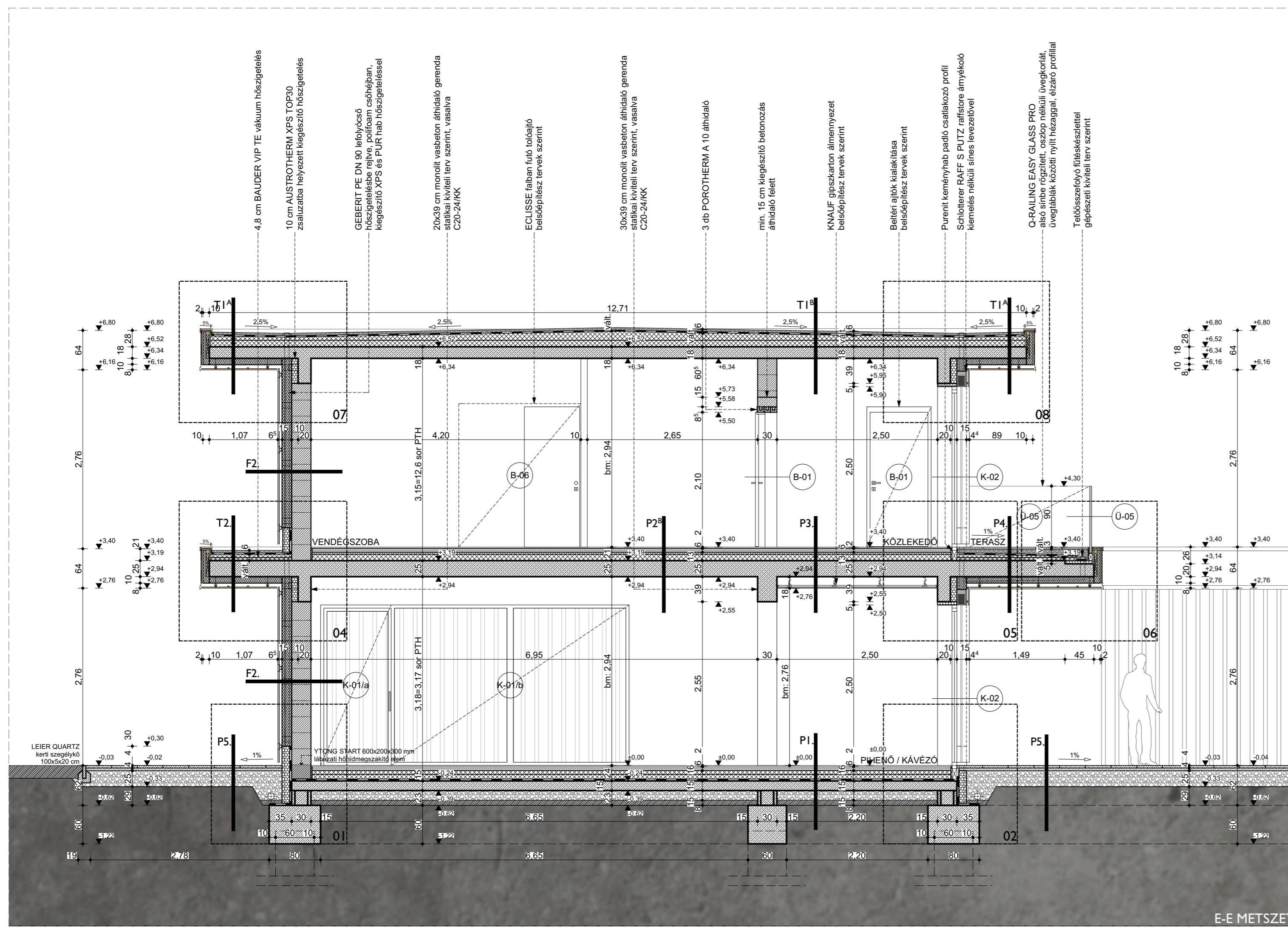
E-E METSZET
