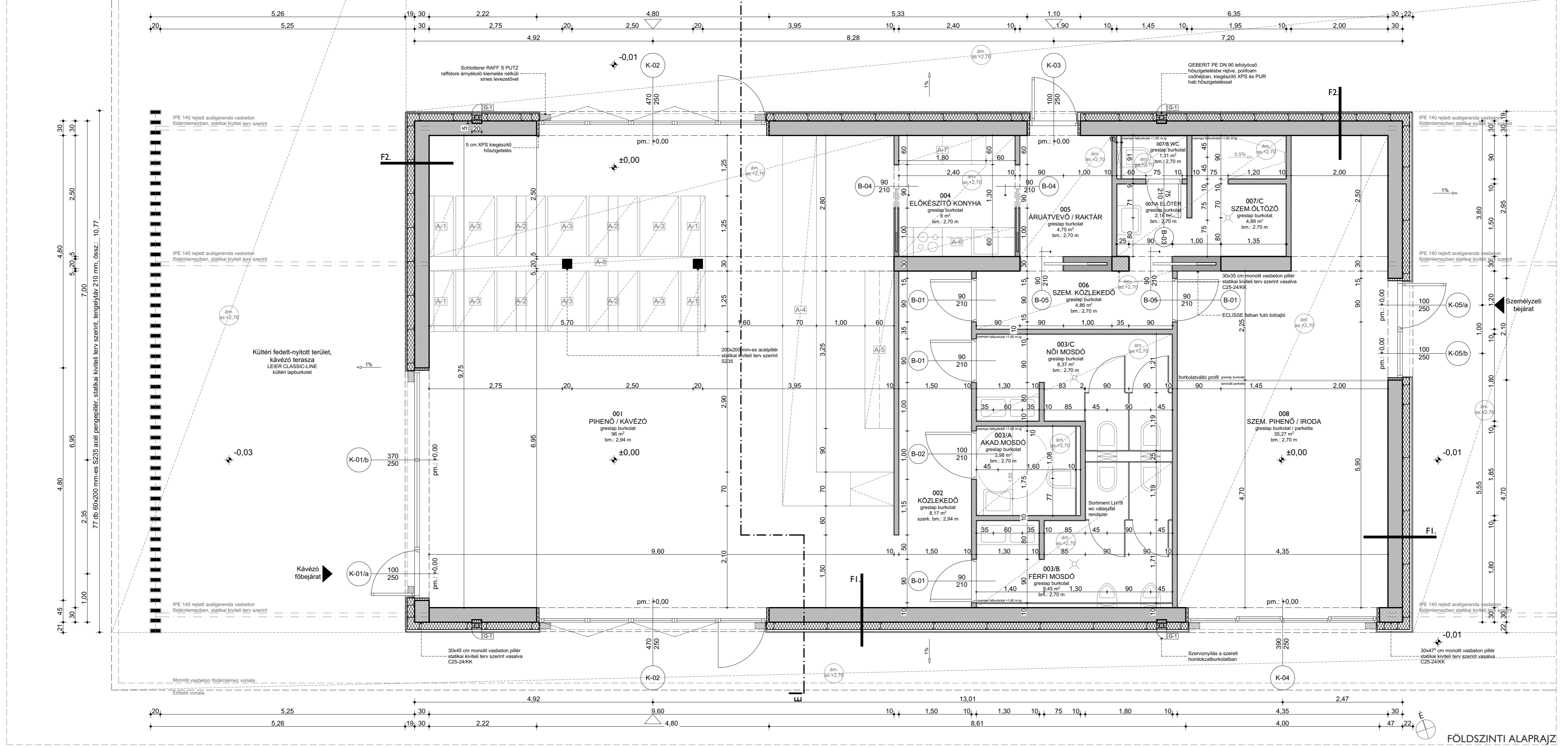
FÖLDSZINTI ALAPRAJZ
