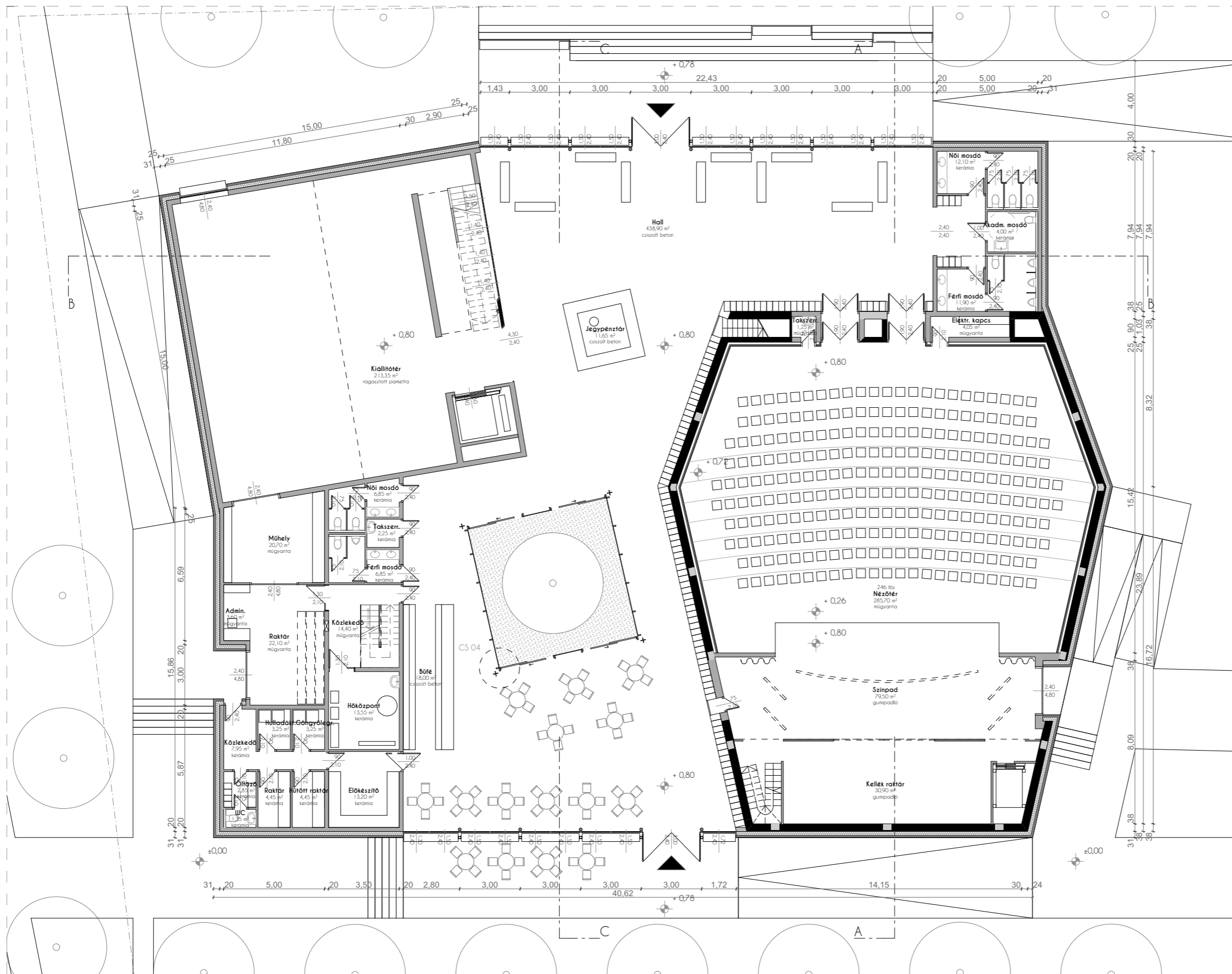
FÖLDSZINTI ALAPRAJZ
