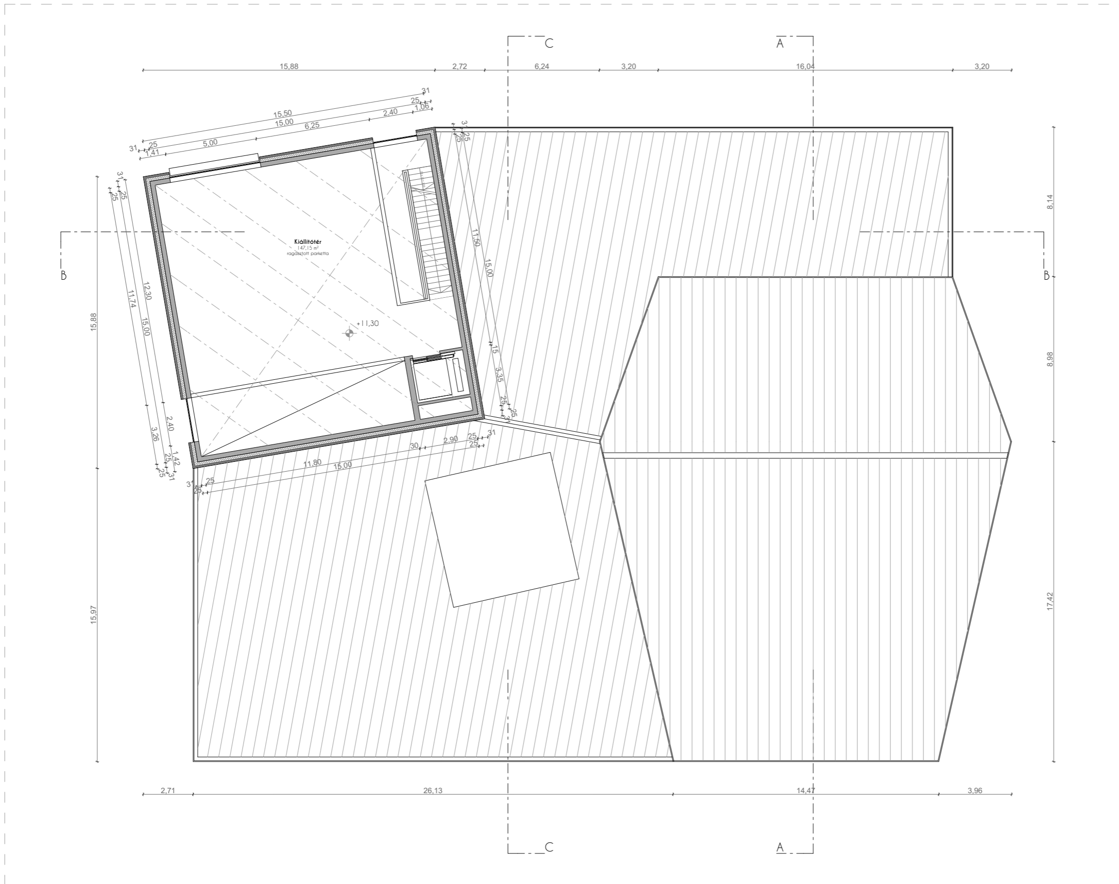
3. EMELETI ALPRAJZ
