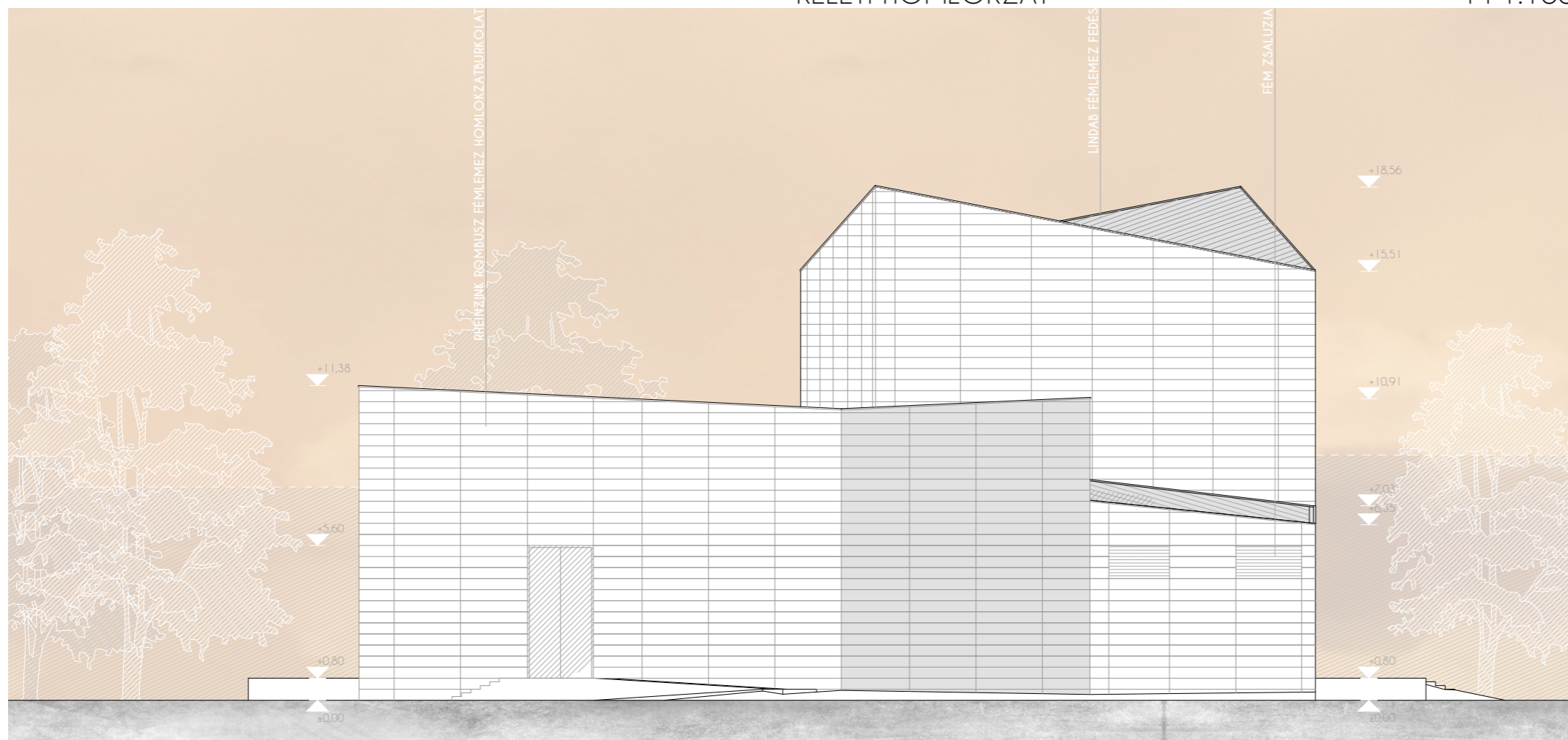
KELETI HOMLOKZAT
