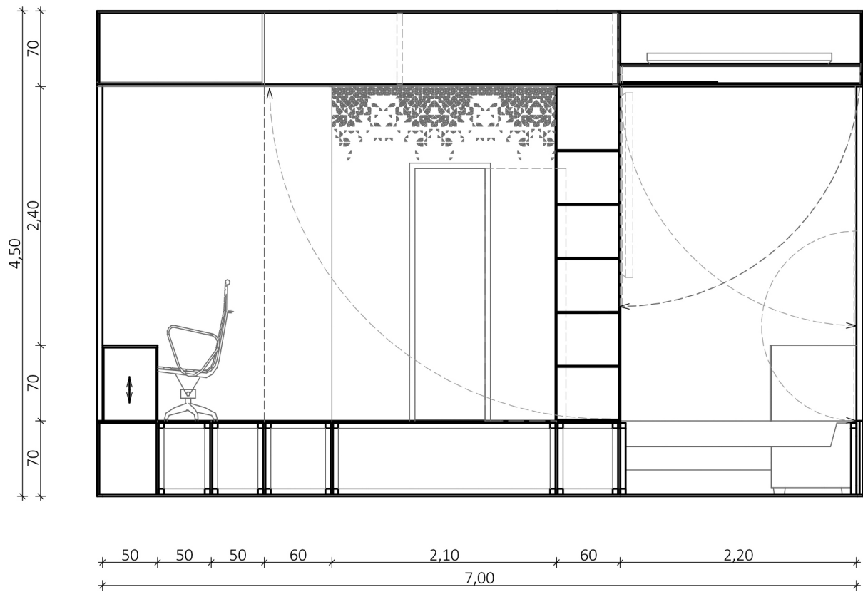
Falnézet és burkolatkiosztás M1:50
