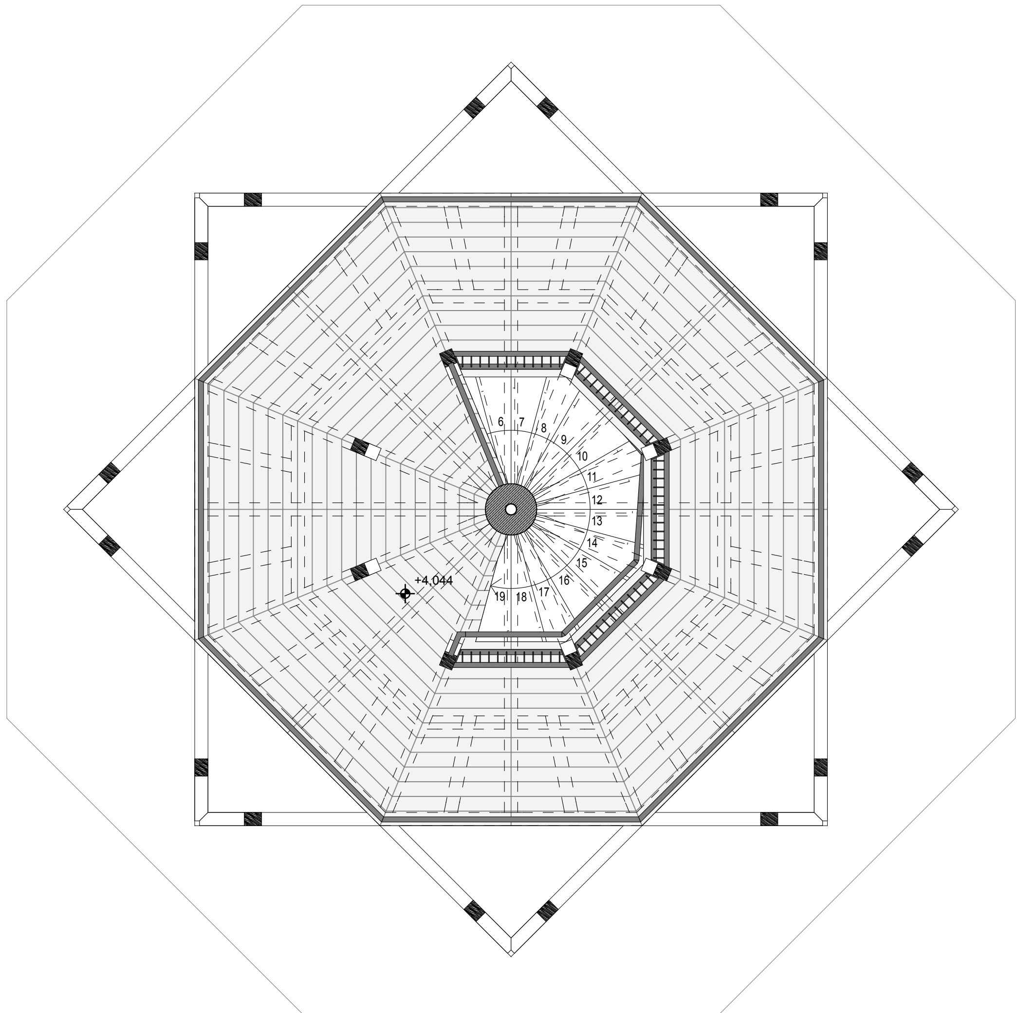
KILÁTÓ SZINTI ALAPRAJZ
