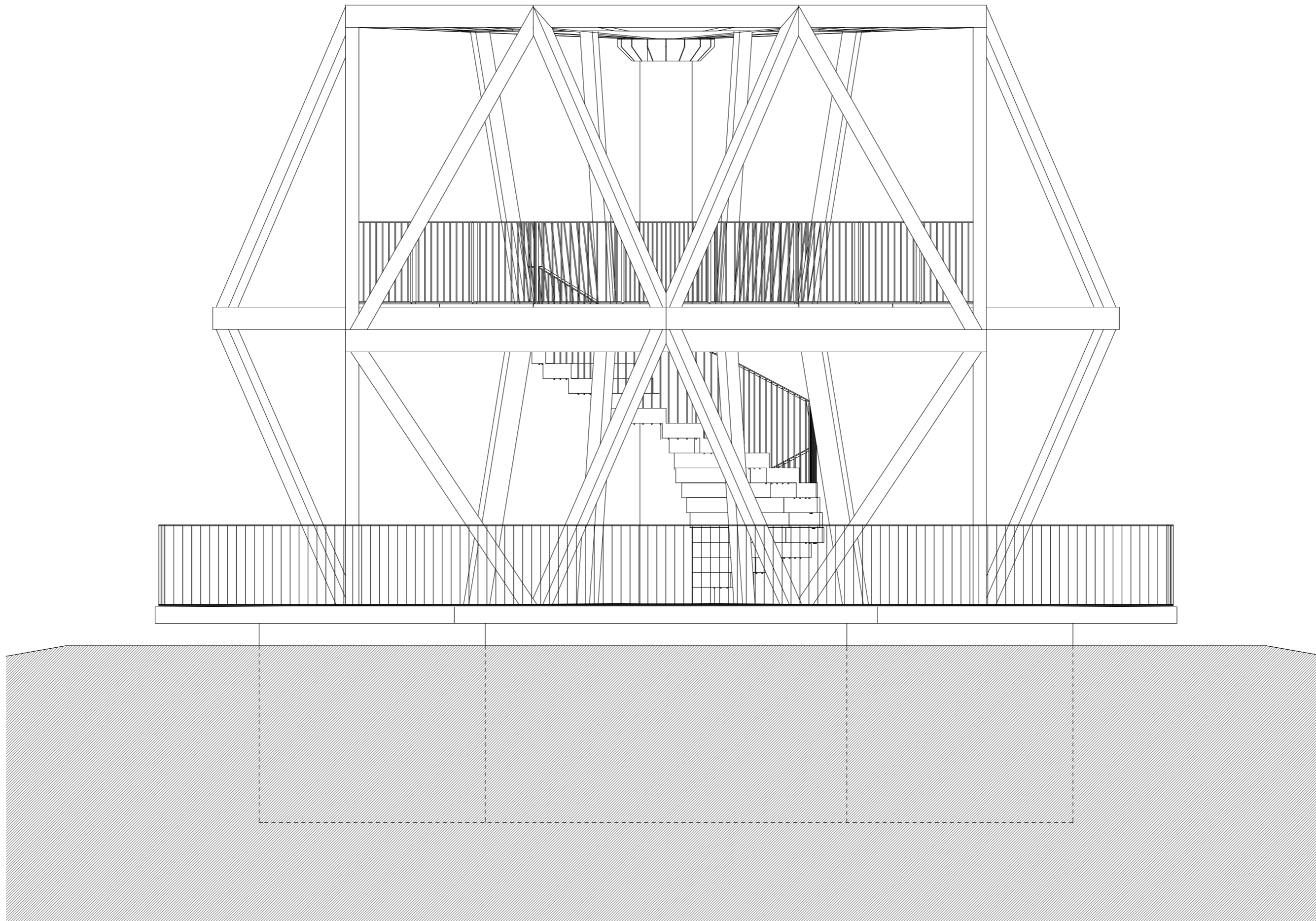
ÉSZAK-NYUGATI HOMLOKZAT
