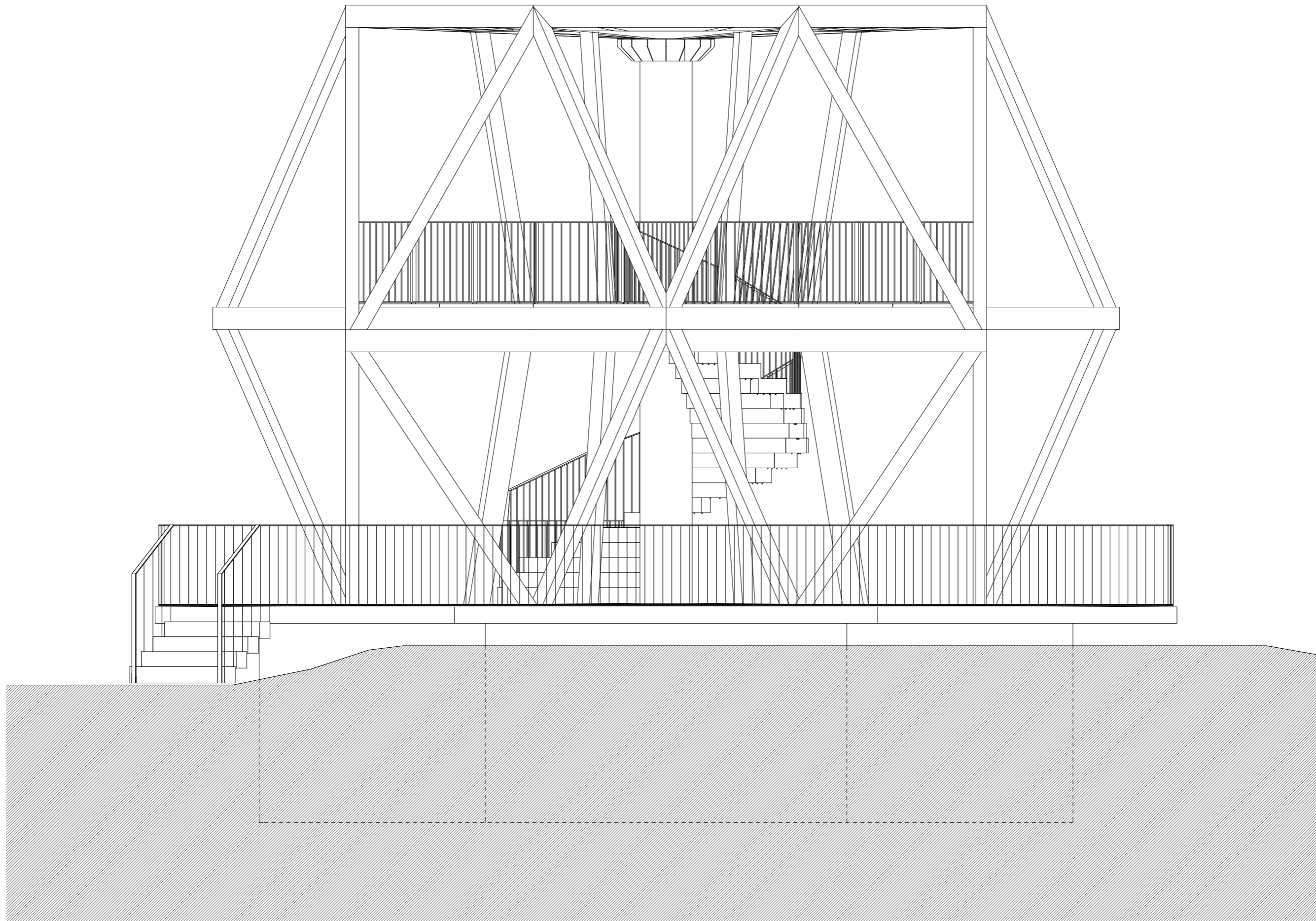
ÉSZAK-KELETI HOMLOKZAT
