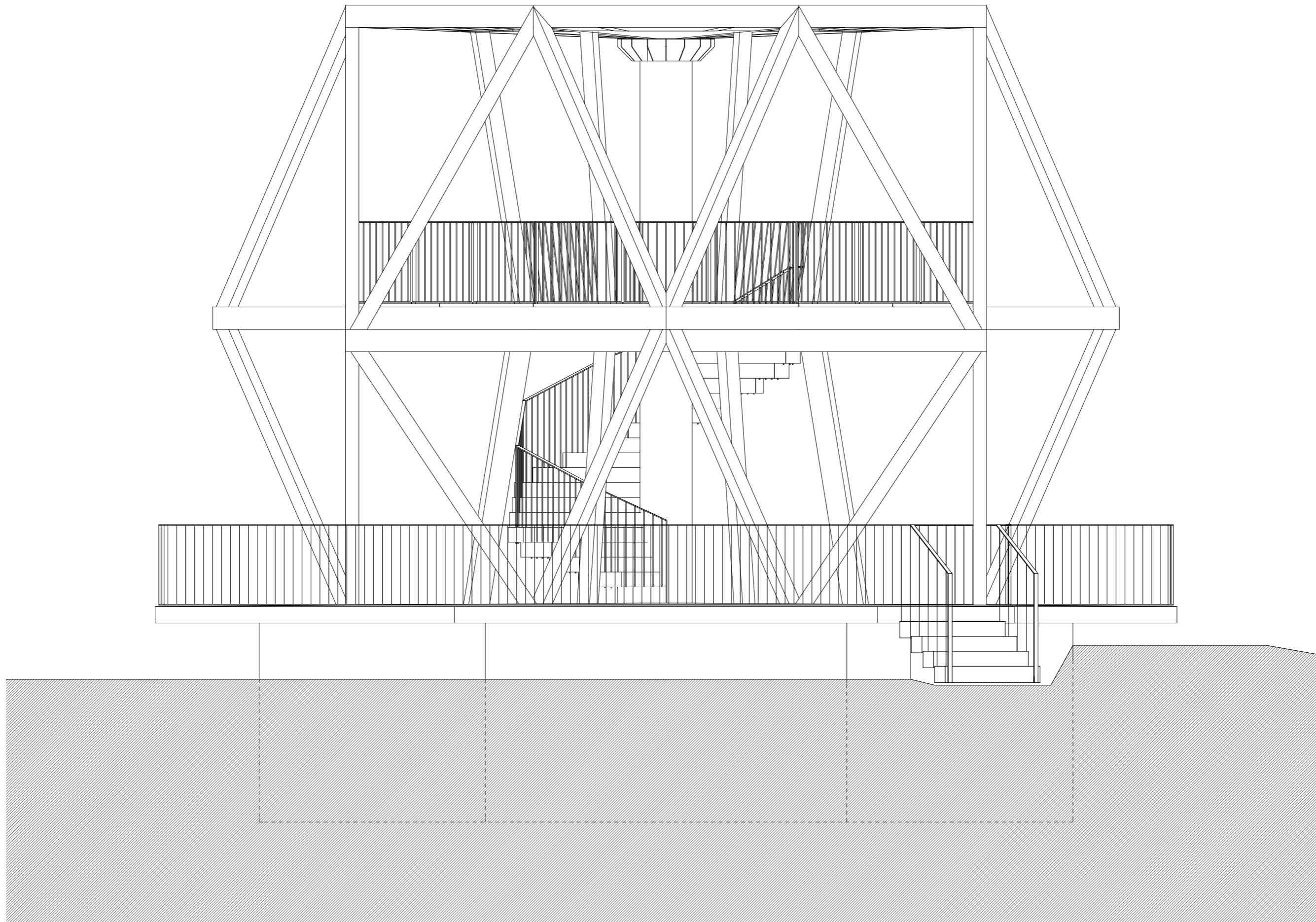
DÉL-KELETI HOMLOKZAT
