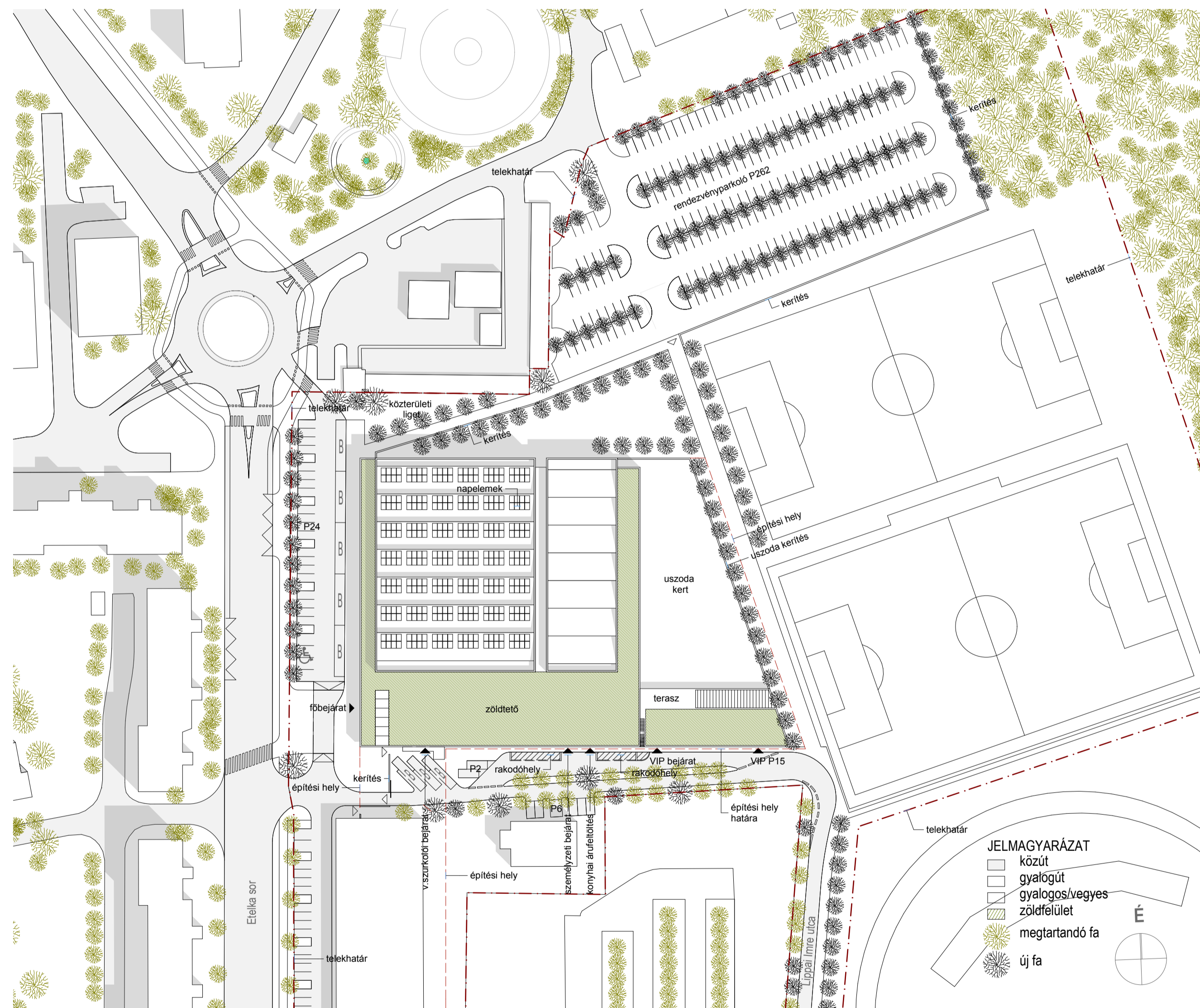
HELYSZÍNRAJZ 1/1000
