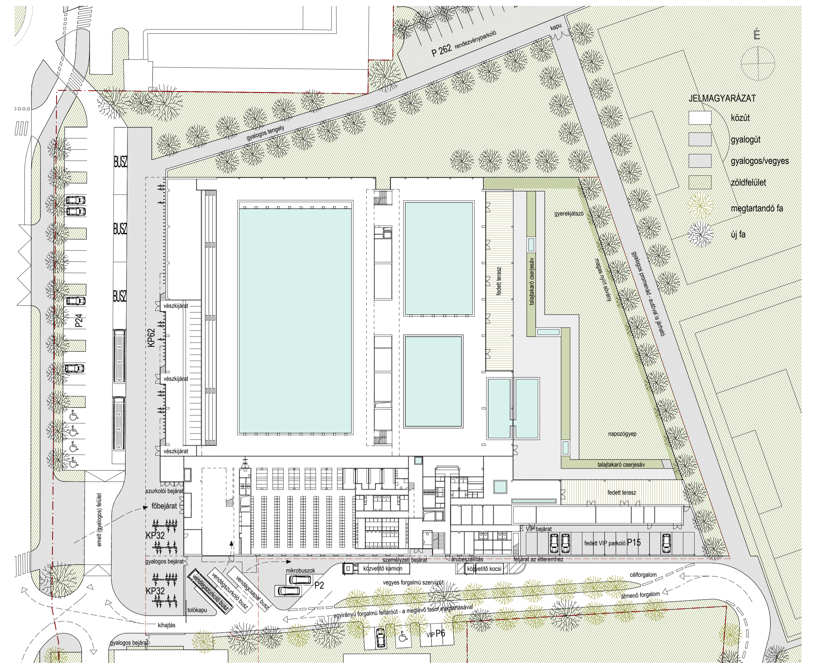
KÖRNYEZETI TERV ÉS FORGALMI HELYSZÍNRAJZ 1/500
