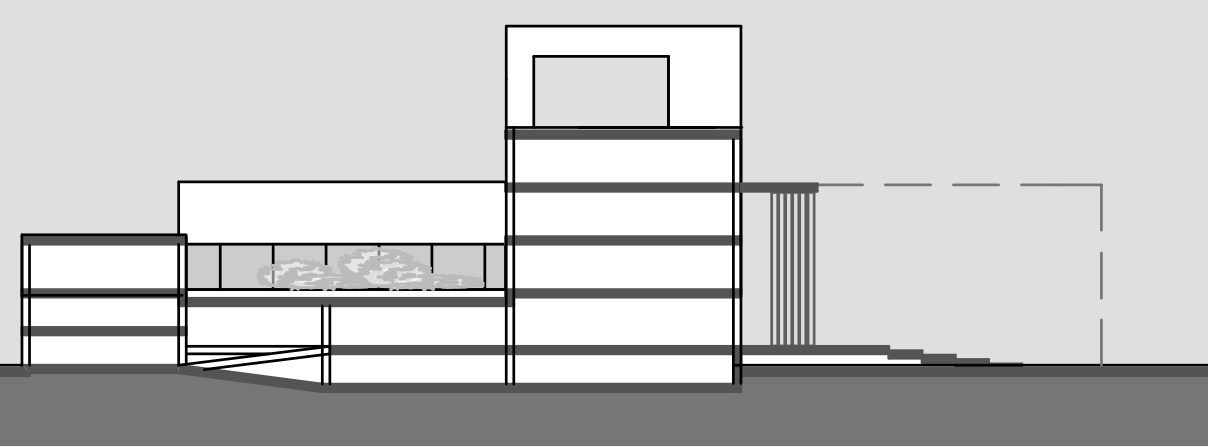
METSZET
