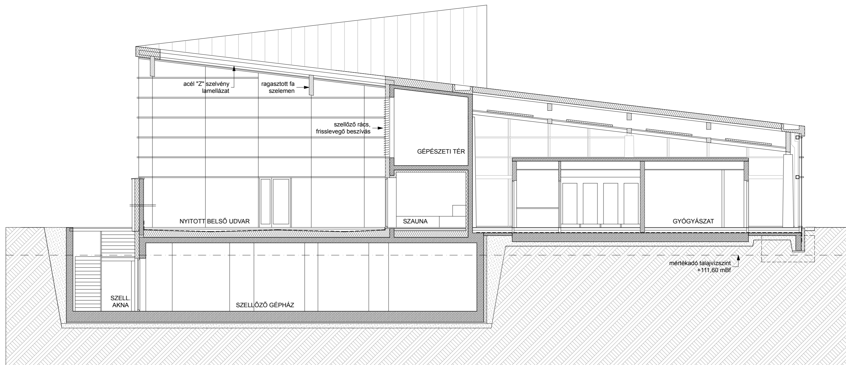
BB METSZET
