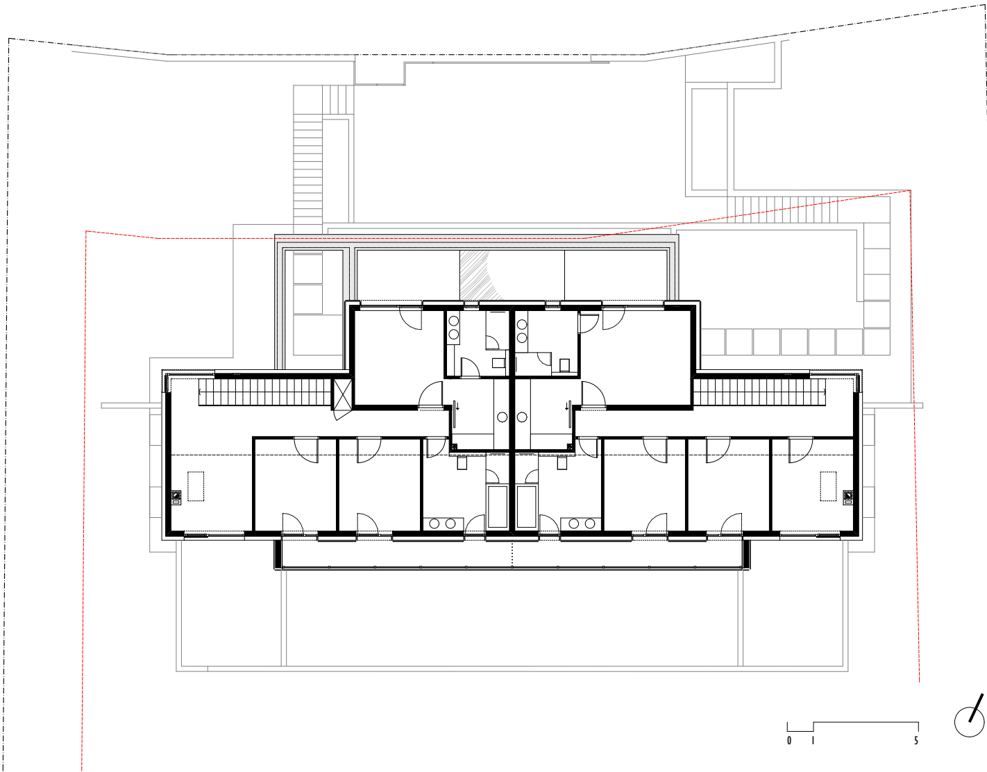
EMELETI ALAPRAJZ
