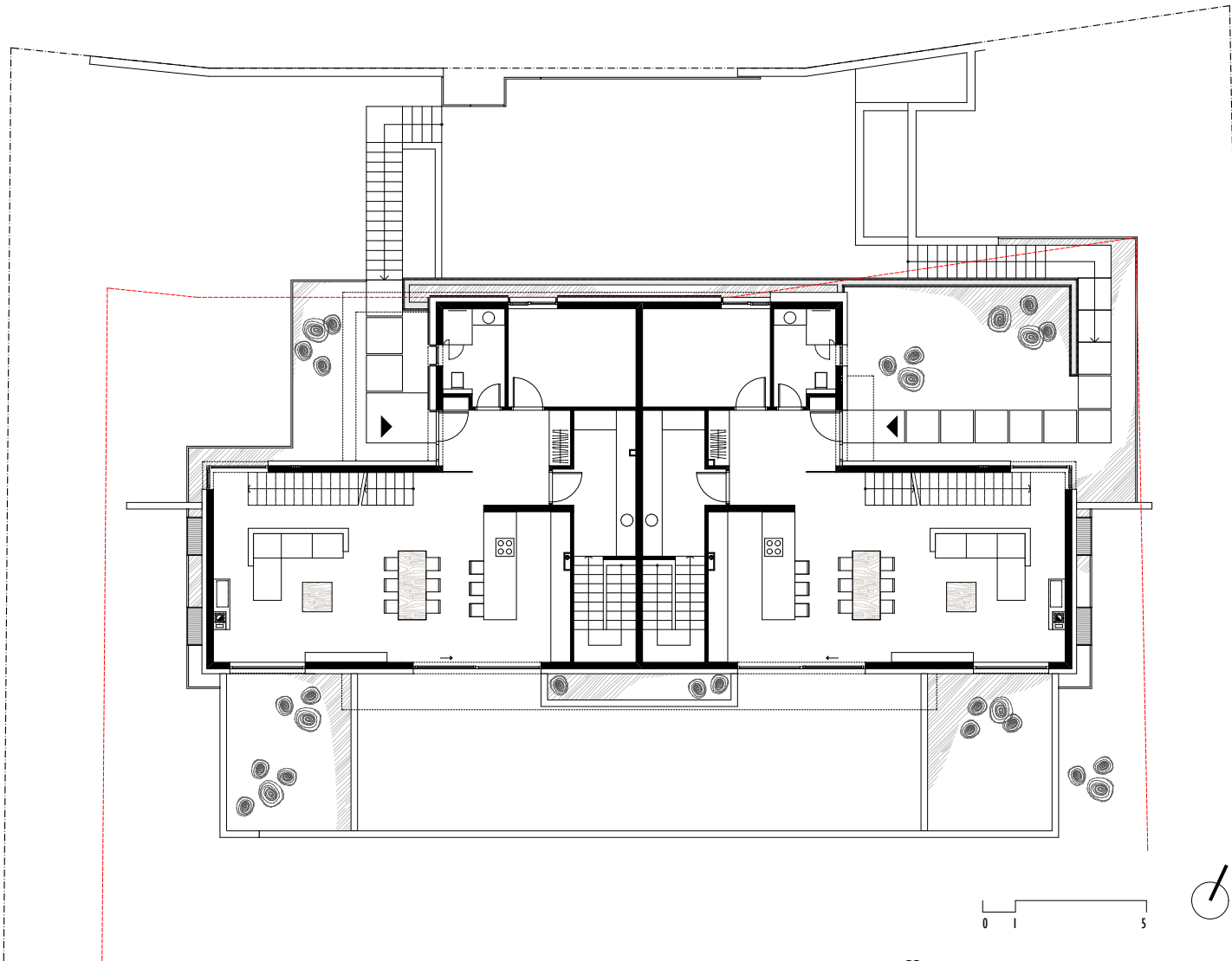
FÖLDSZINTI ALAPRAJZ
