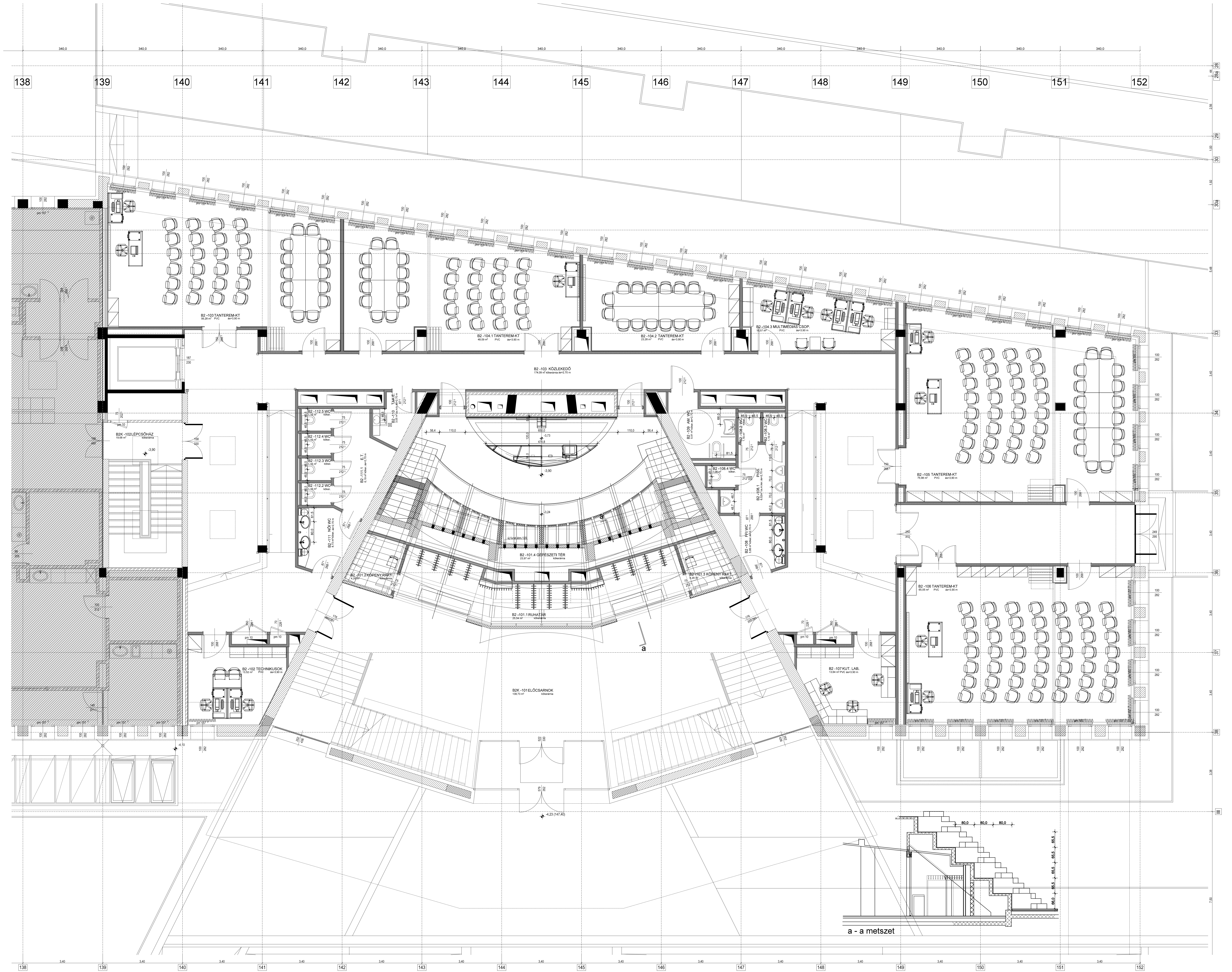
OKTATÁSI SZÁRNY - MÉLYFÖLDSZINT - BERENDEZÉSI ALAPRAJZ
