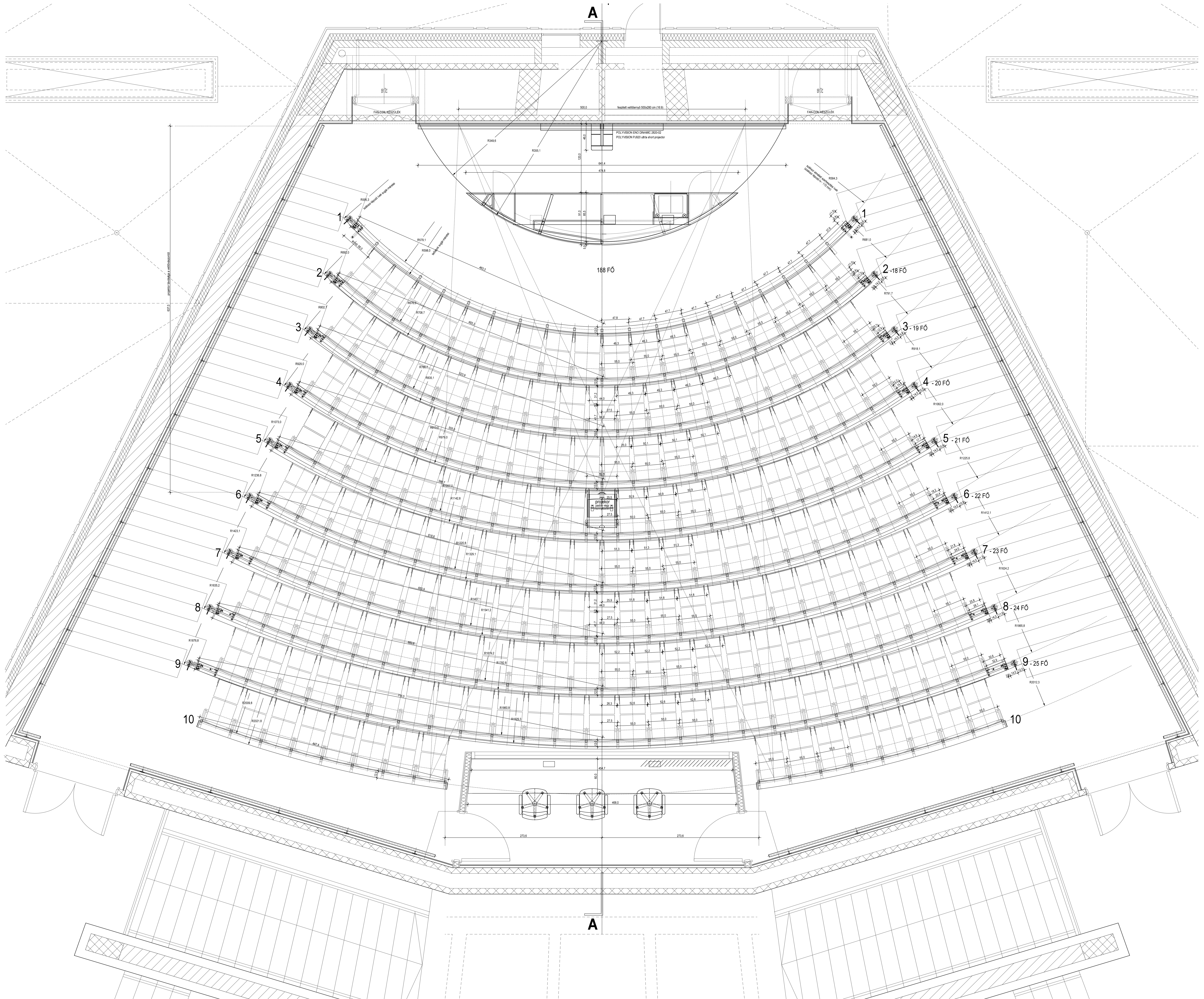
NAGYELŐADÓ ALAPRAJZA
