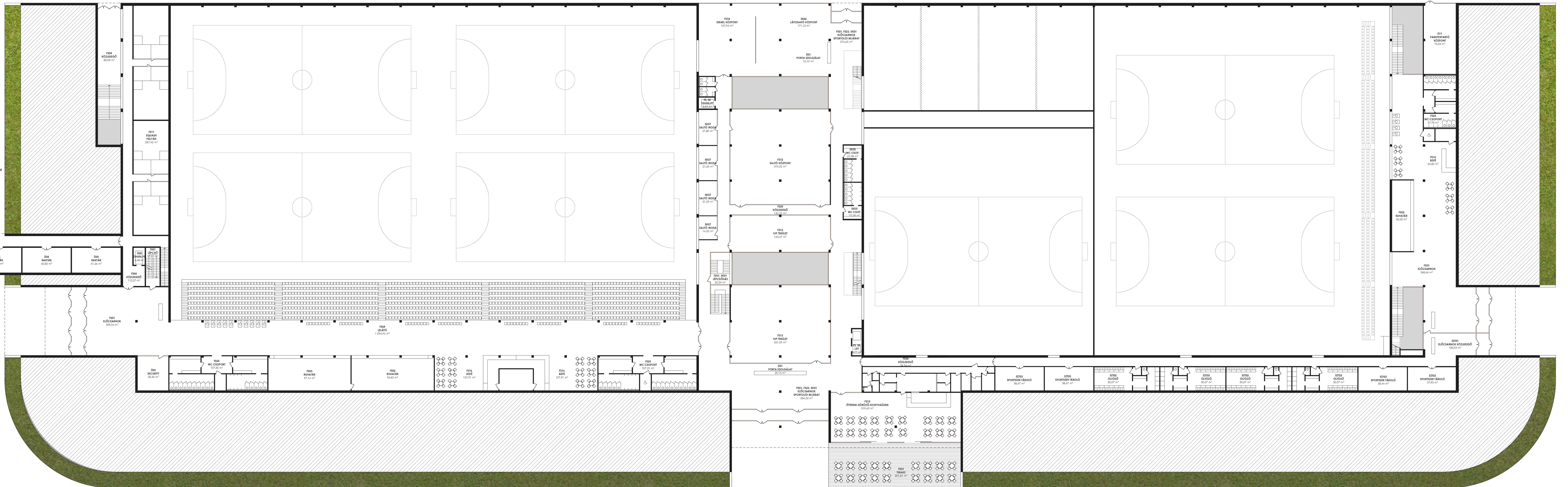
FÖLDSZINTI ALAPRAJZ
