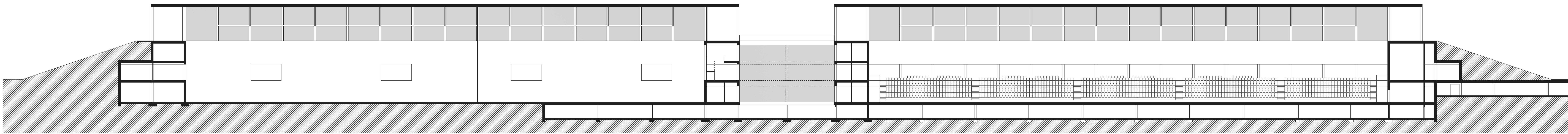
HOSSZMETSZET
