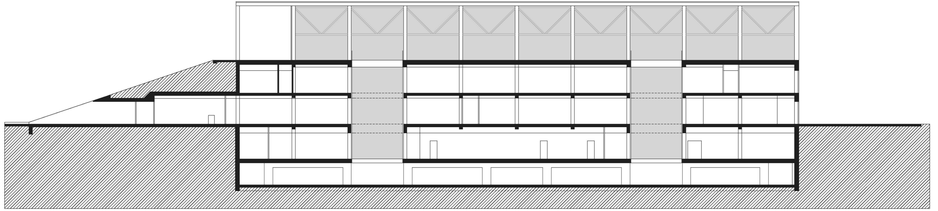
CSARNOKOK KÖZÖTTI KERESZTMETSZET
