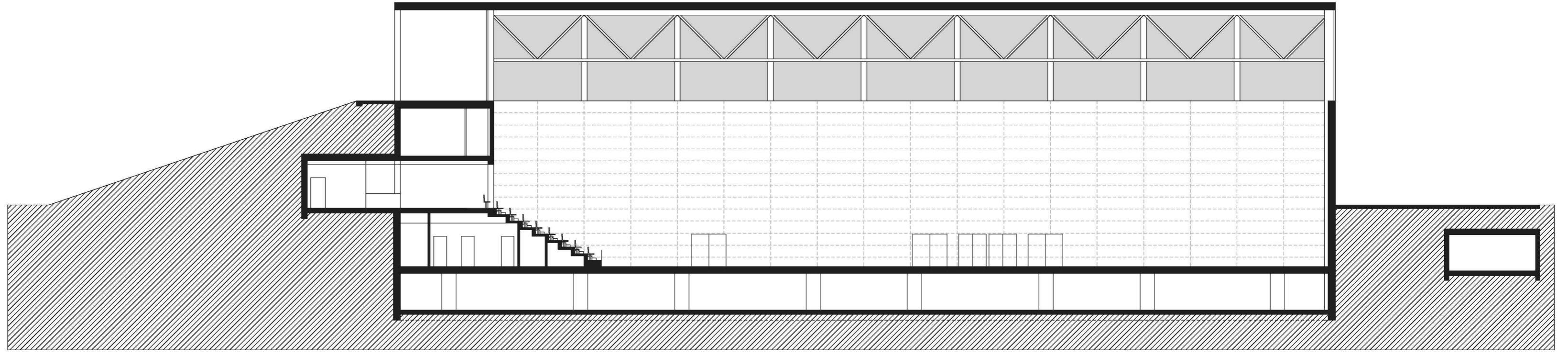
I. CSARNOK KERESZTMETSZETE
