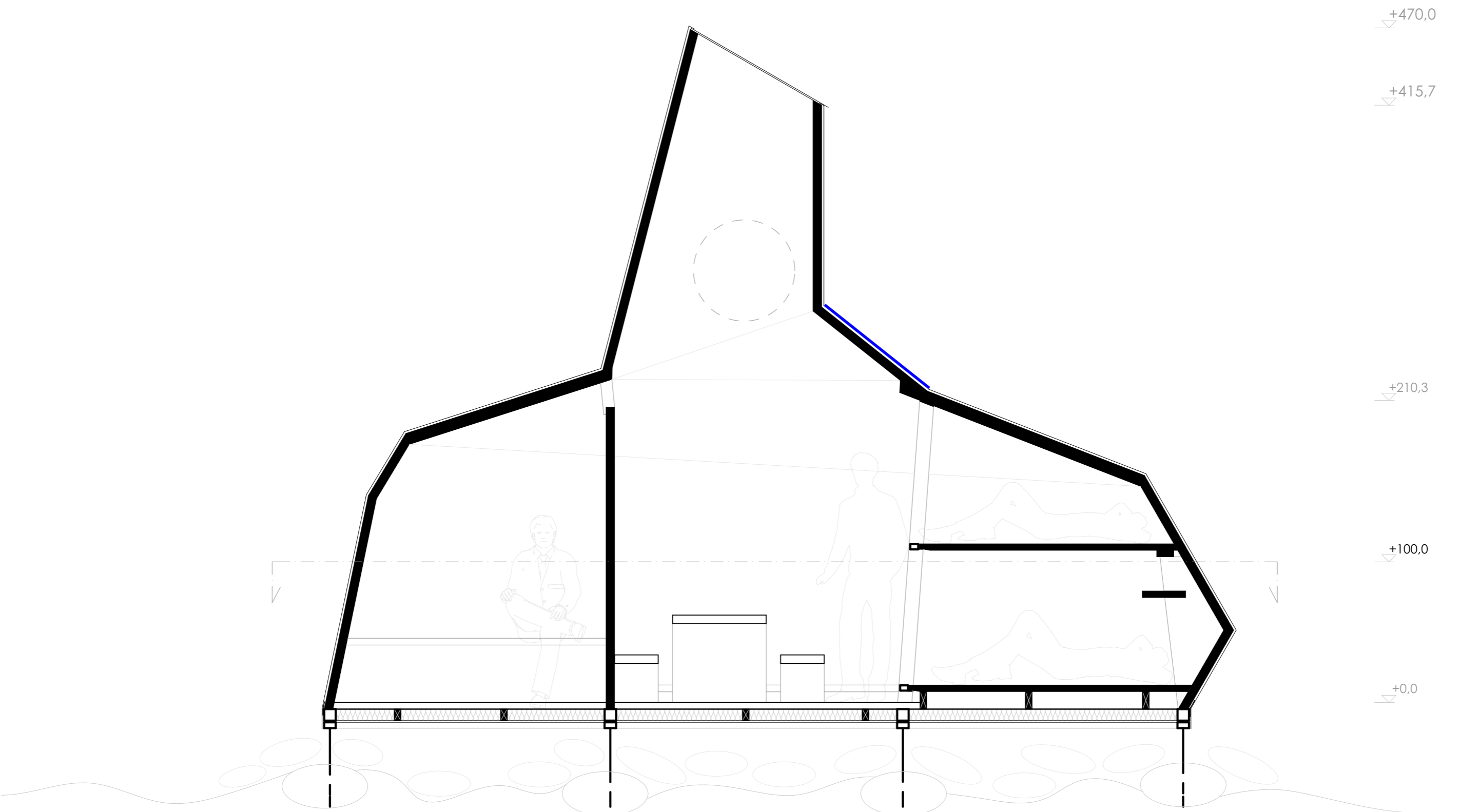
SECTIUNE A-A¹
