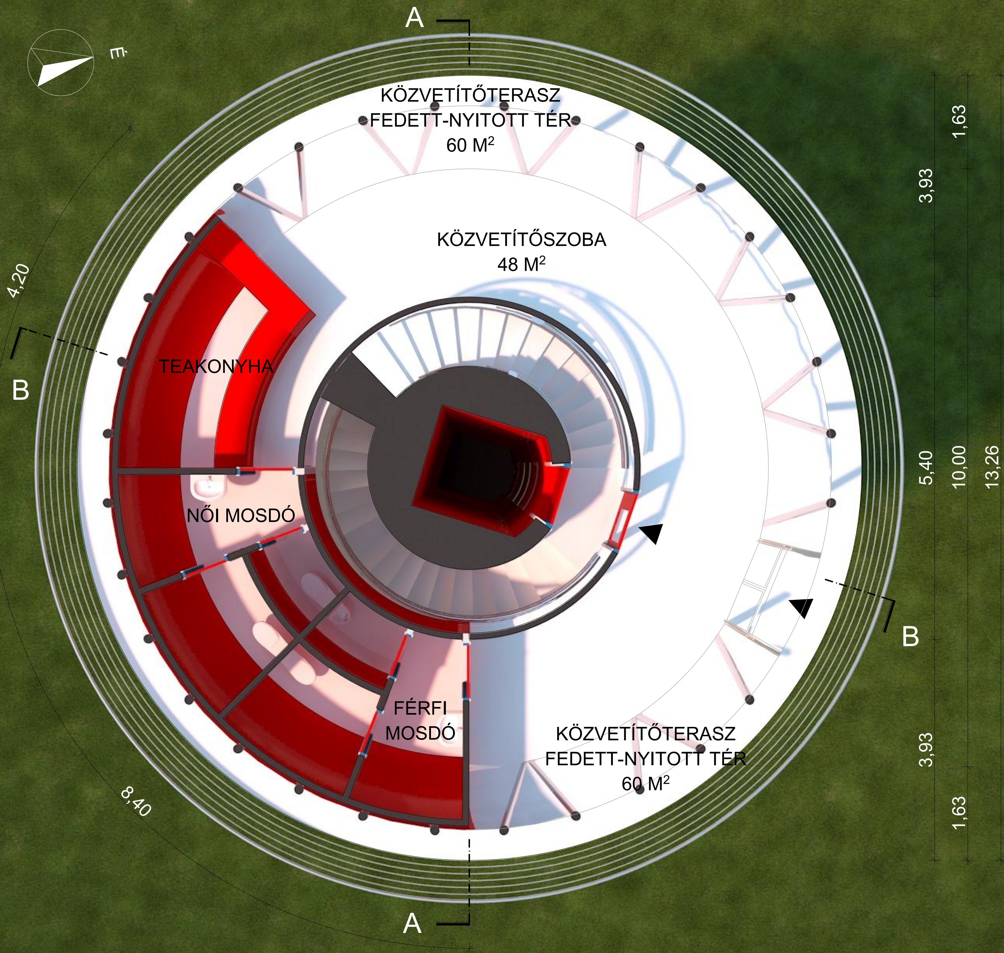
5. EMELETI ALAPRAJZ
