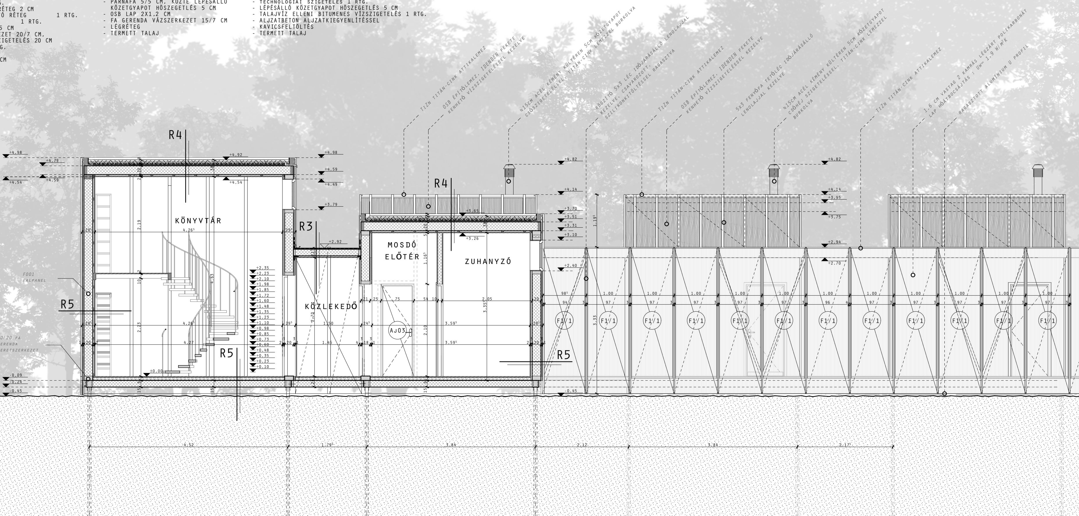
METSZET RÉSZLET M 1:50
