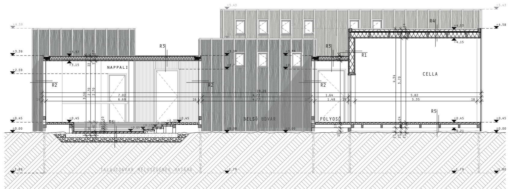
M-01 METSZET M 1:100
