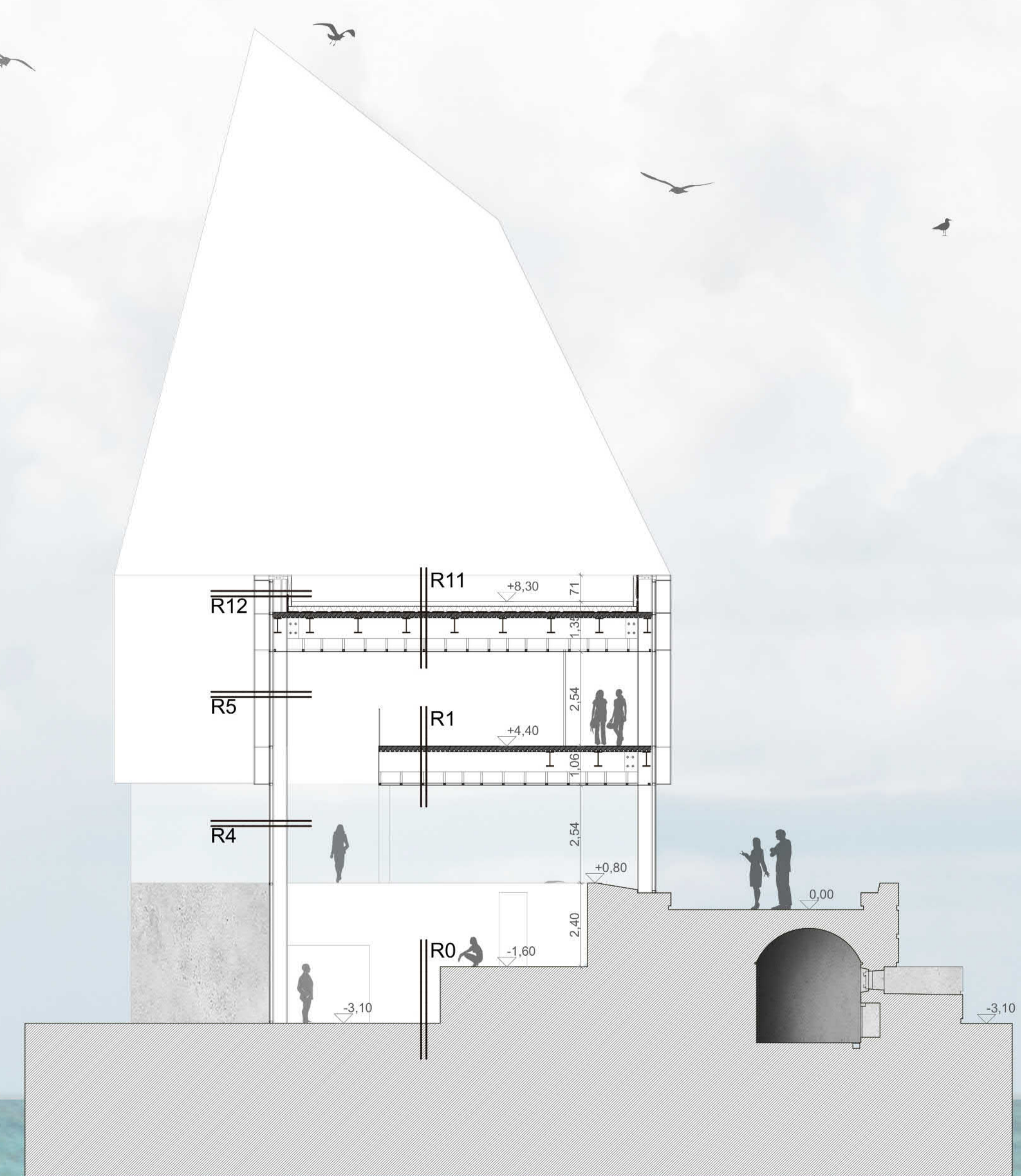
I-I METSZET M1:100
