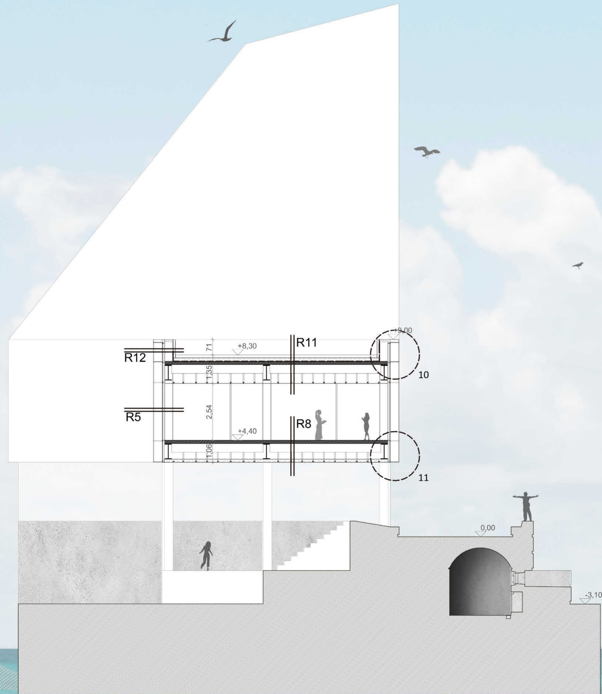
G-G METSZET M1:100
