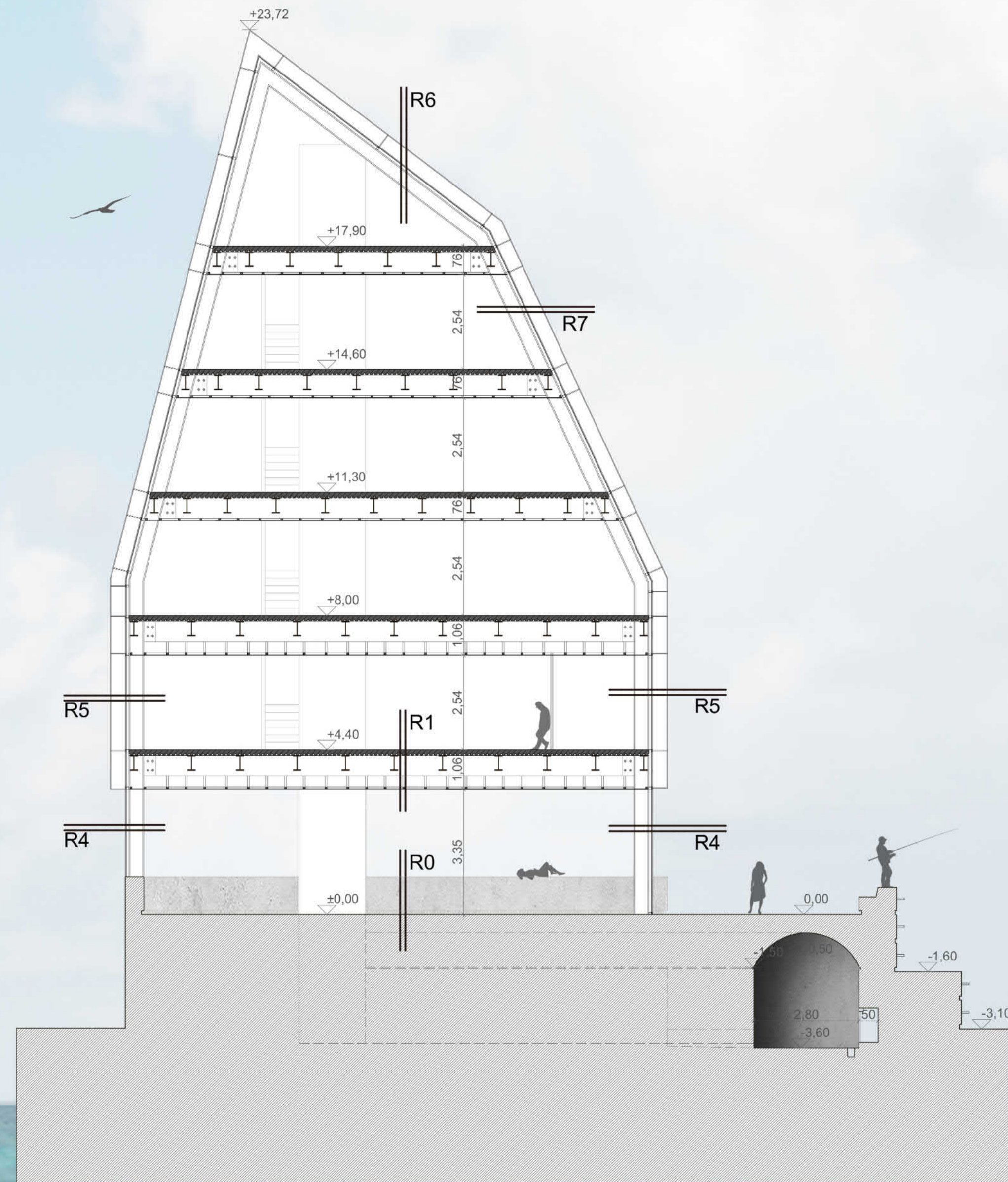
H-H METSZET M1:100
