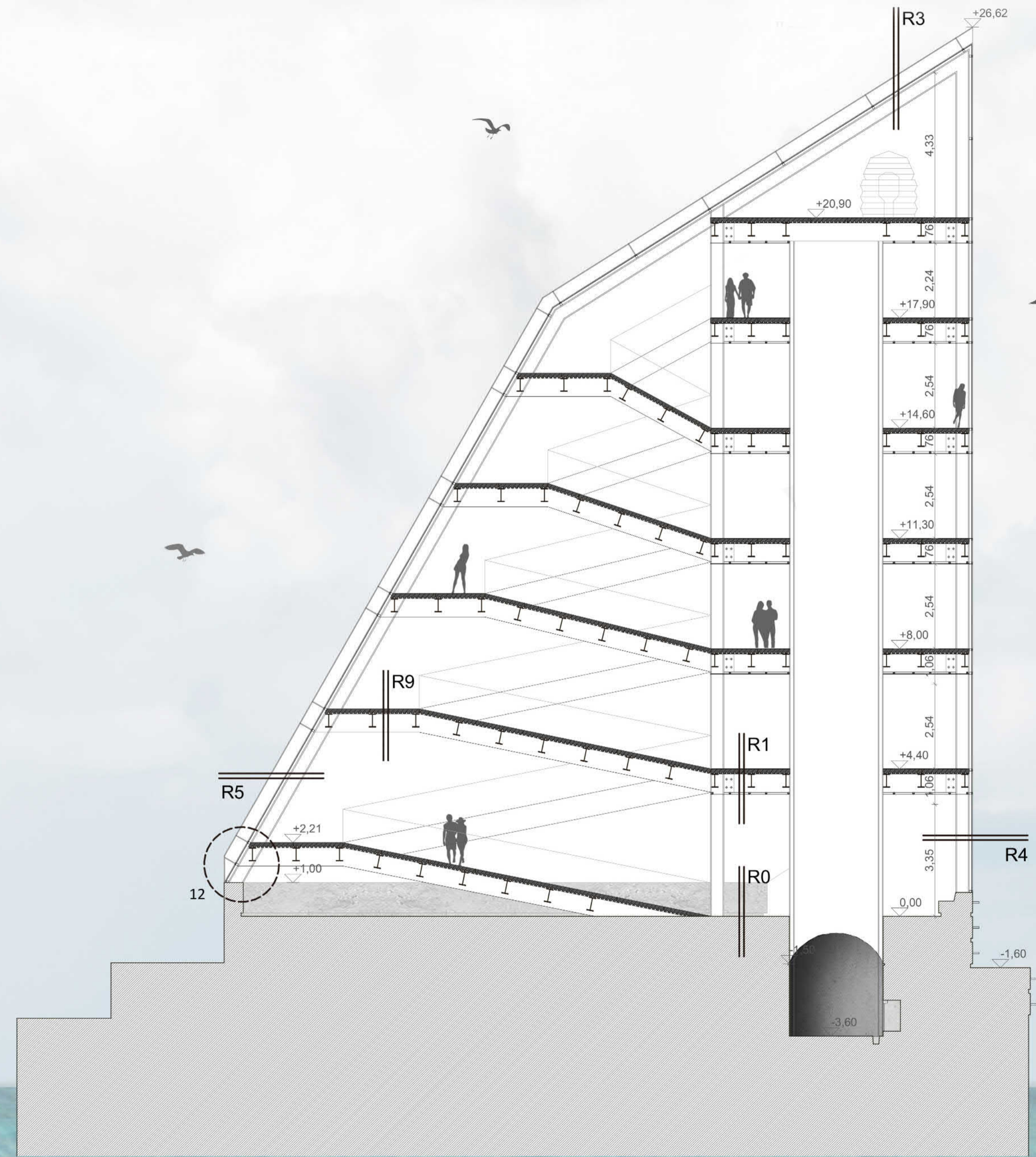
L-L METSZET M1:100
