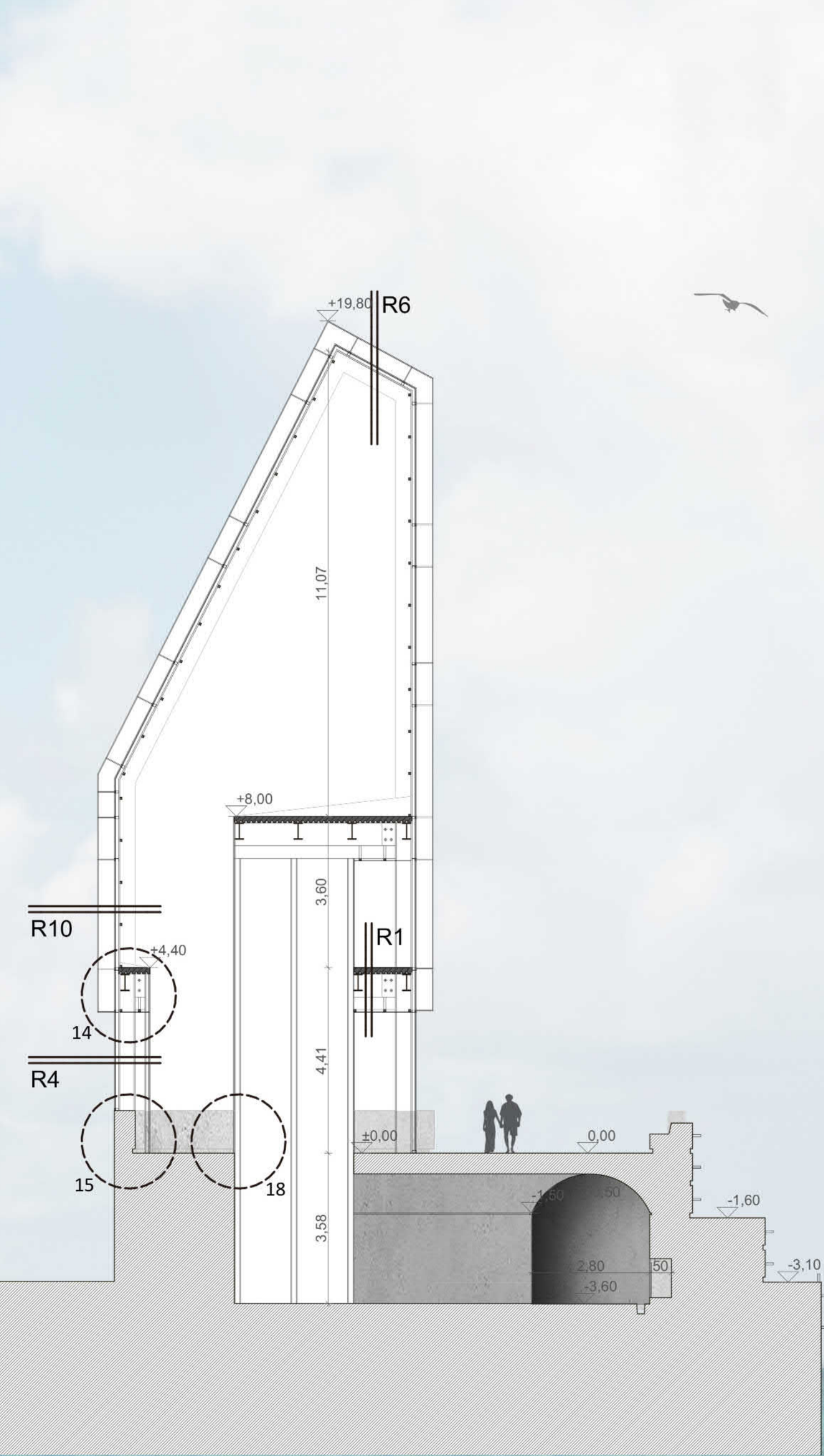
K-K METSZET M1:100
