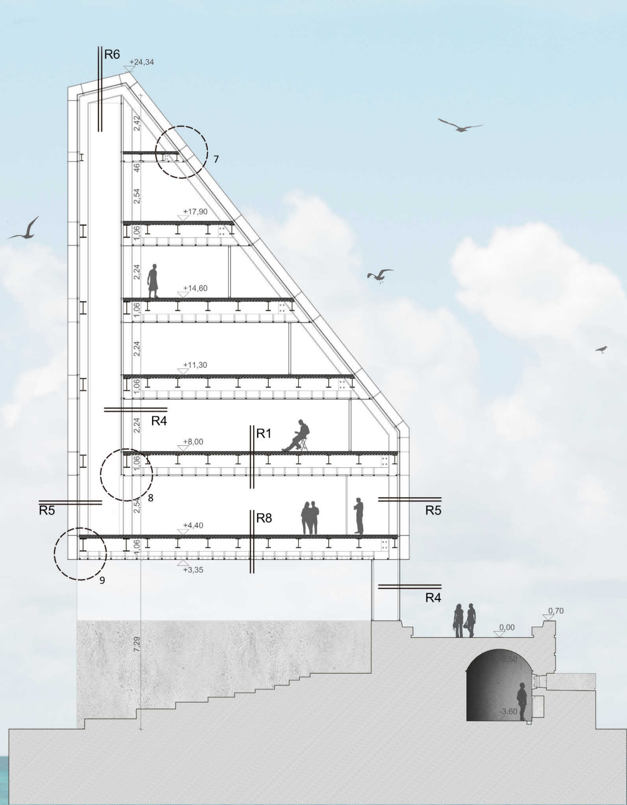
J-J METSZET M1:100
