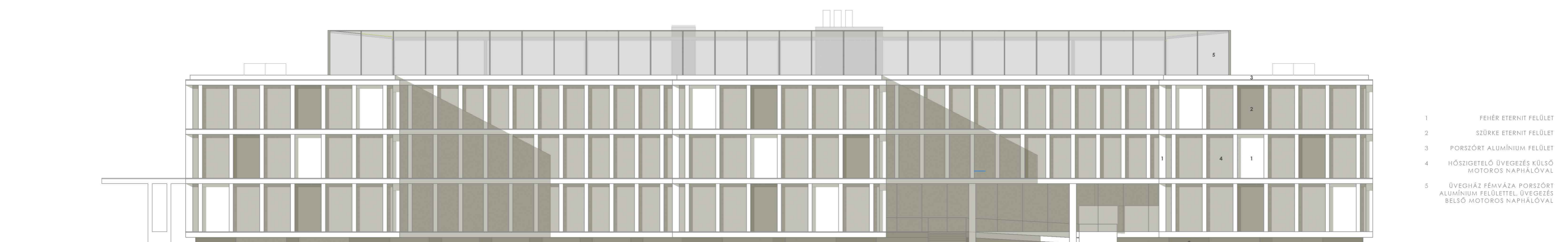
C-C JELŰ METSZET
