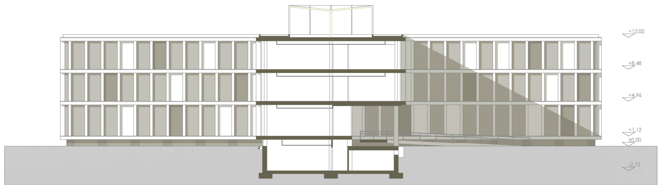
A-A JELŰ METSZET
