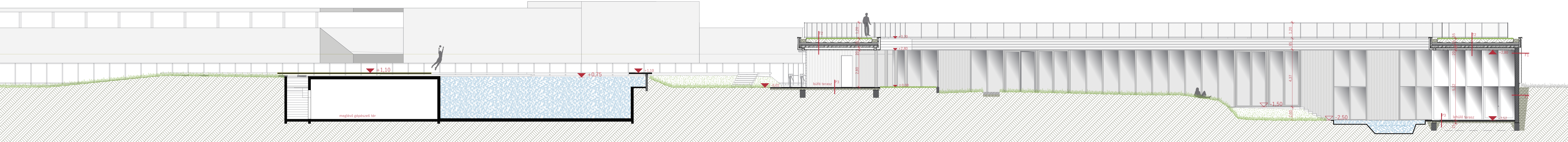
F-F METSZET
