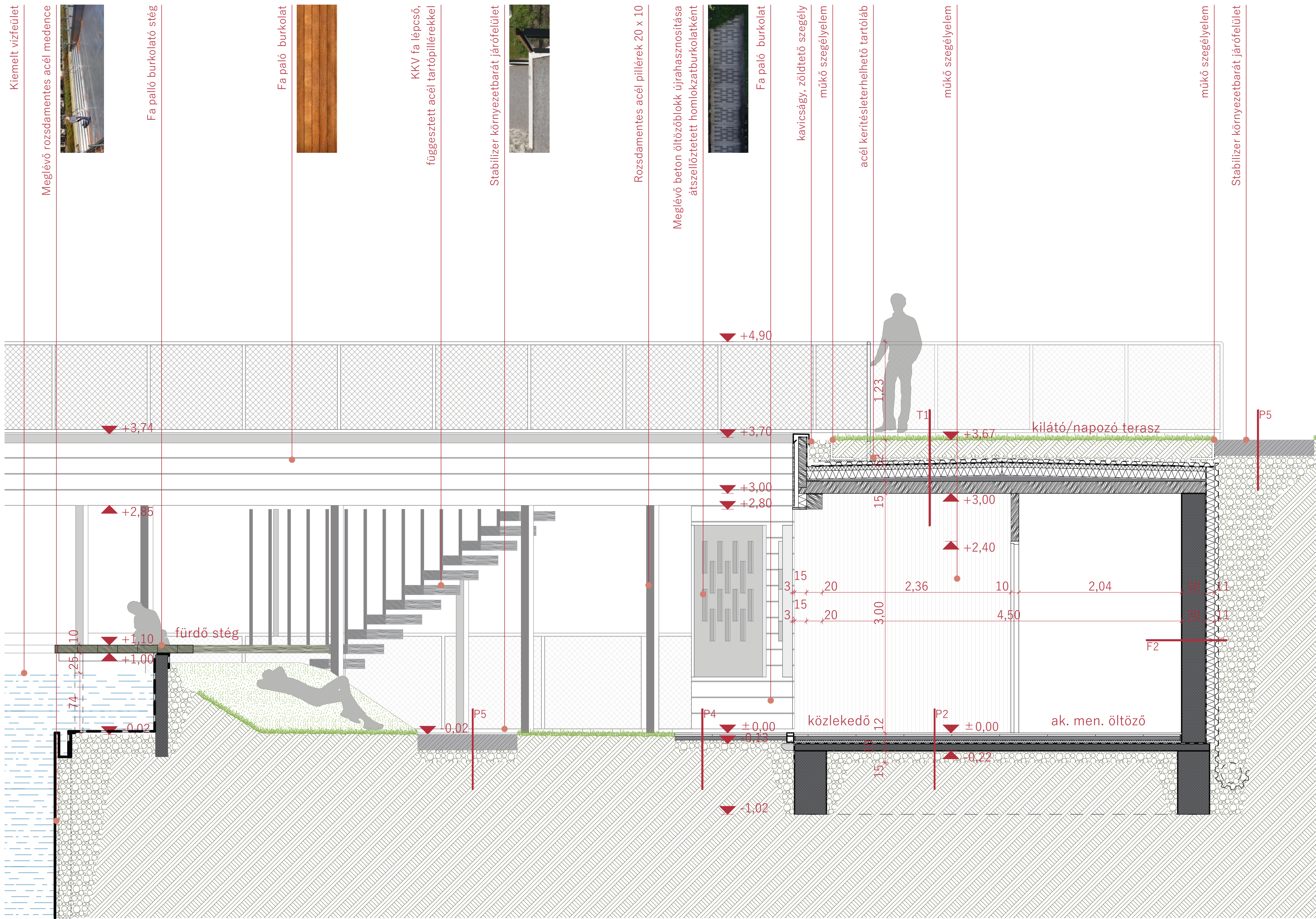
E-E FŐFALMETSZET
