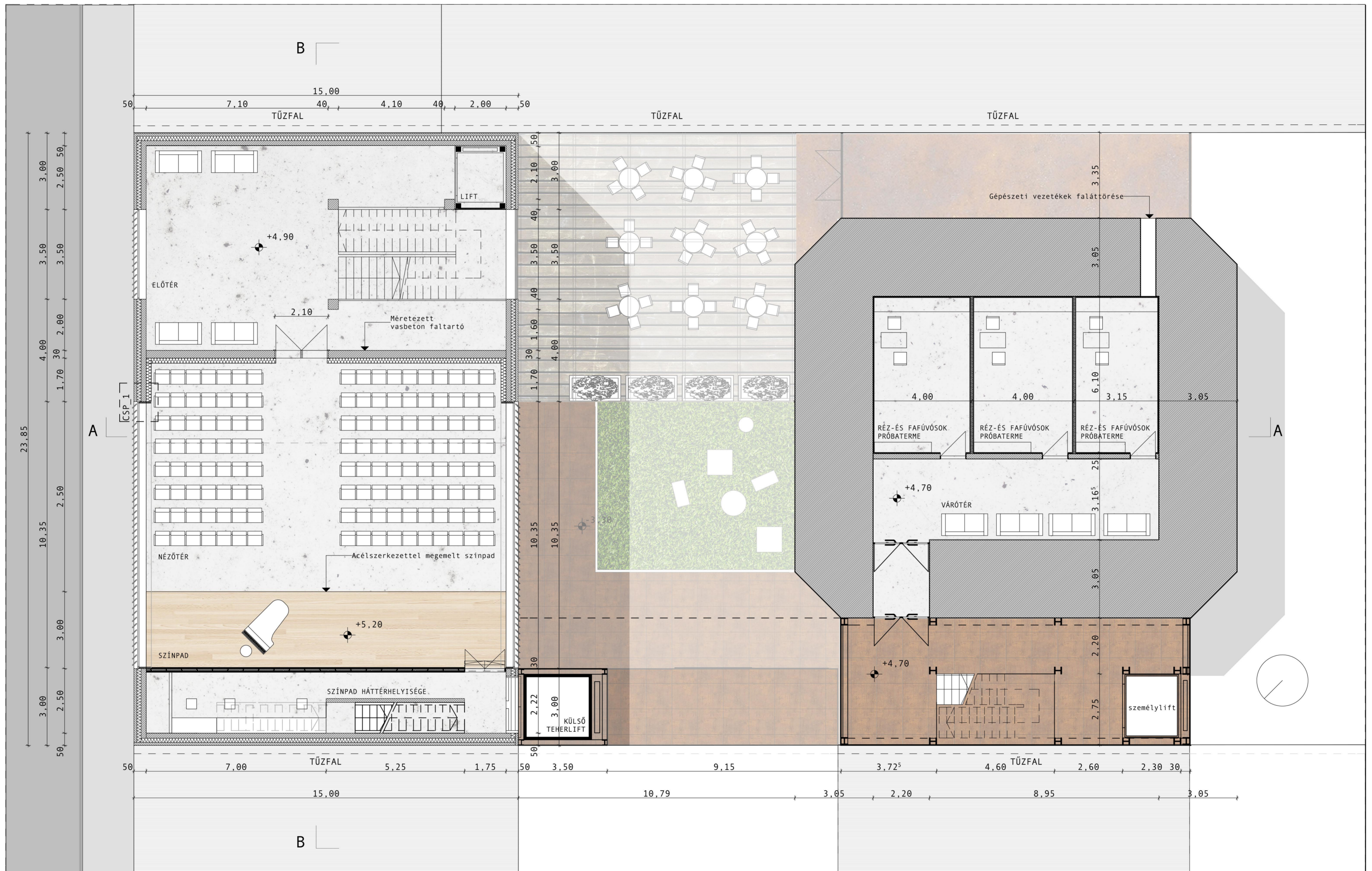
1. EMELETI ALAPRAJZ _ M = 1:100
