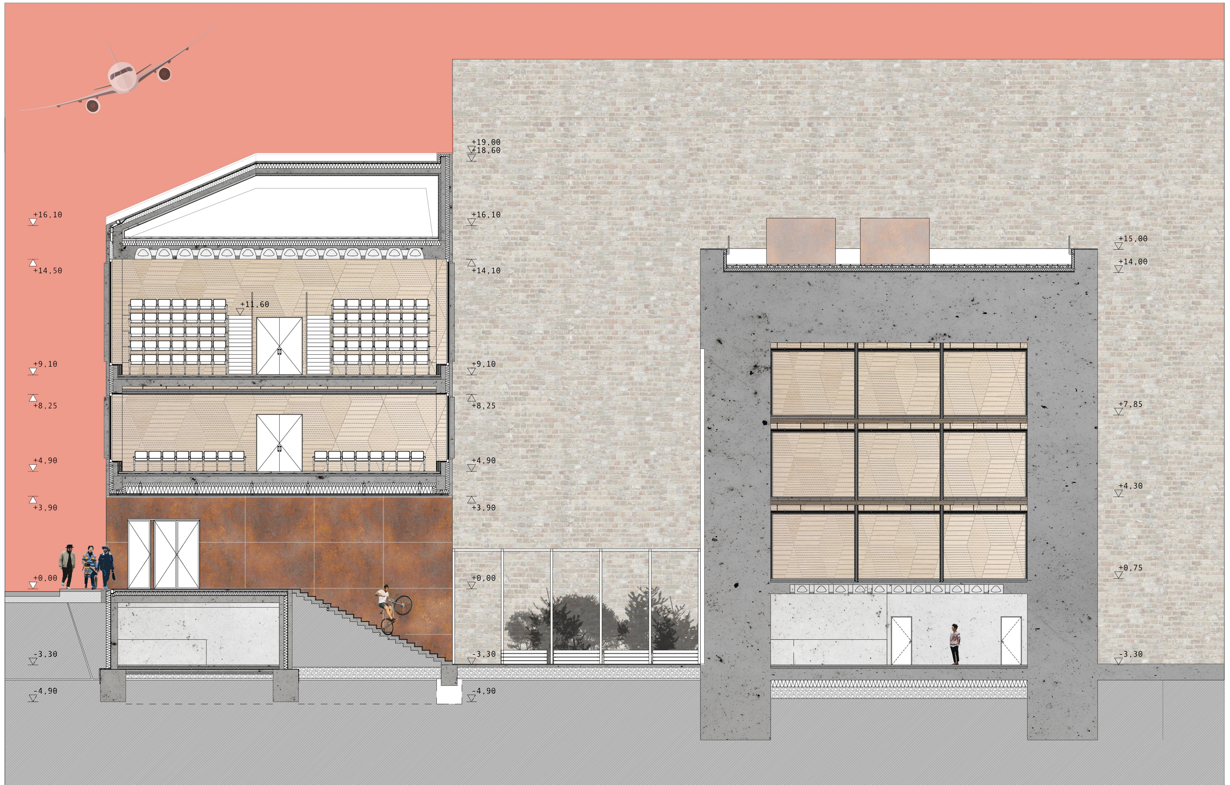
A - A METSZET _ M = 1 : 100
